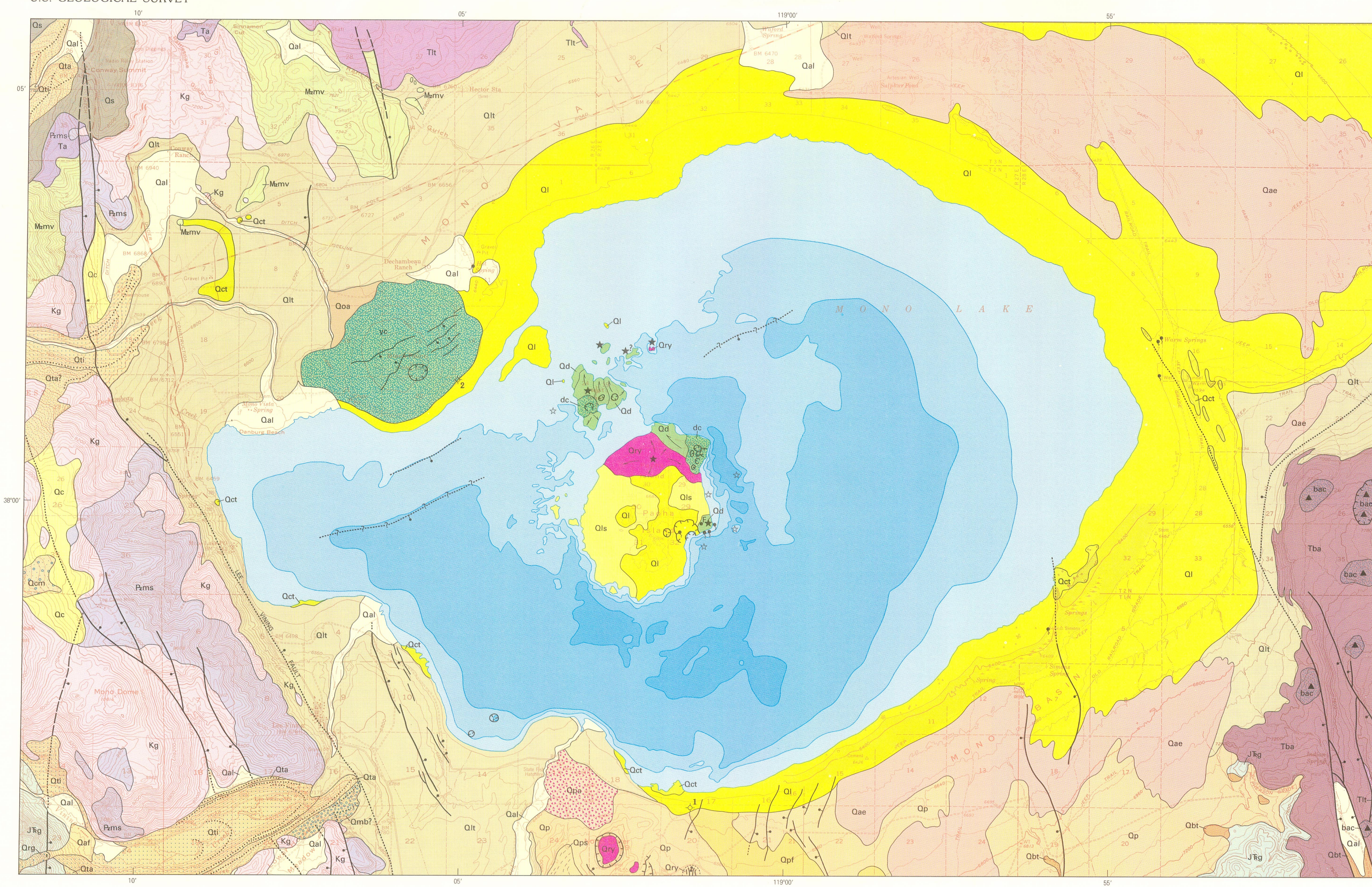
MONO LAKE GEOLOGIC MAP
