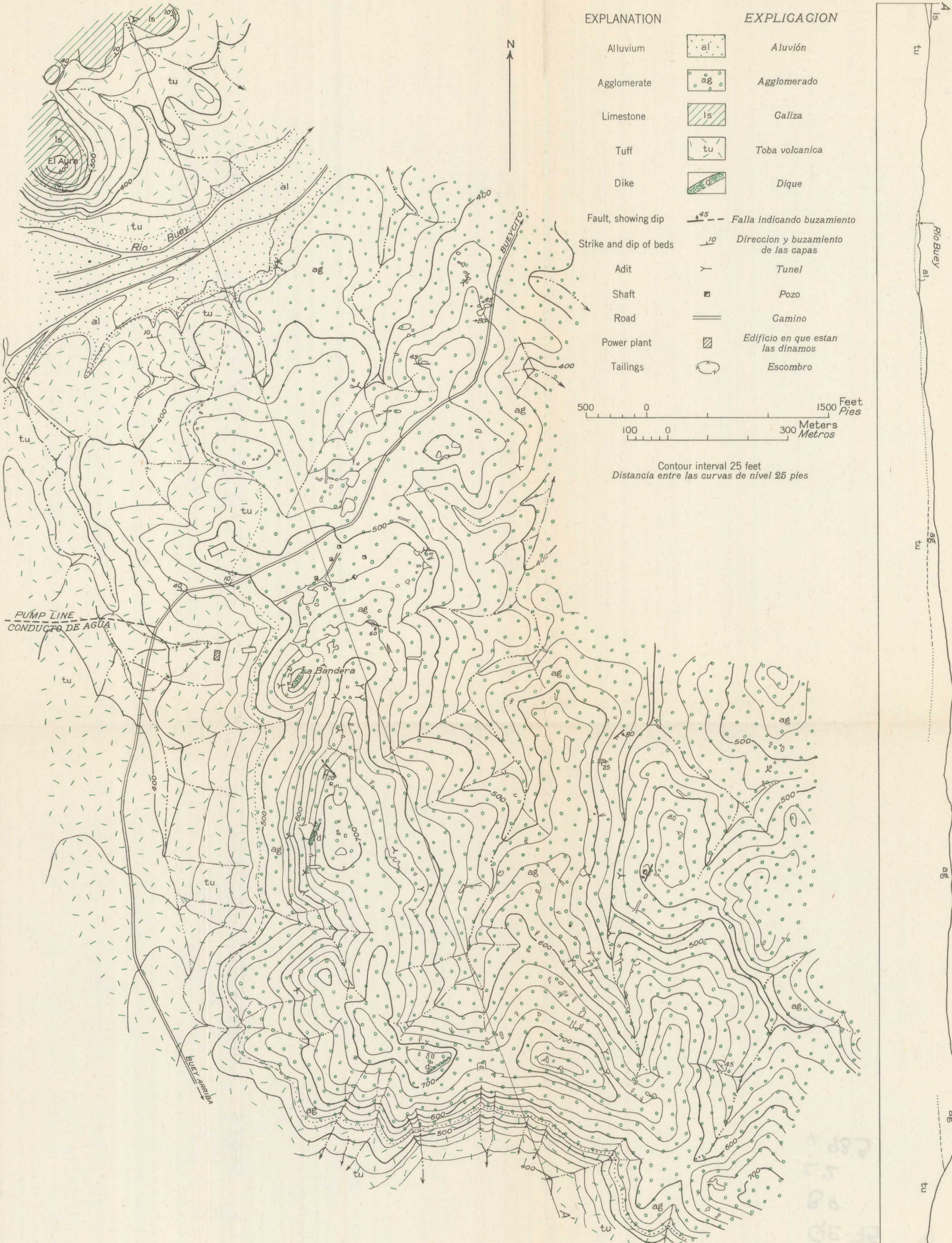
GEOLOGIC MAP AND SECTION OF THE CENTRAL PART OF THE BUEYCITO DISTRICT, ORIENTE PROVINCE, CUBA MAPA GEOLOGICO Y SECCION DE LA PARTE CENTRAL DEL DISTRITO BUEYCITO, PROVINCIA DE ORIENTE, CUBA
