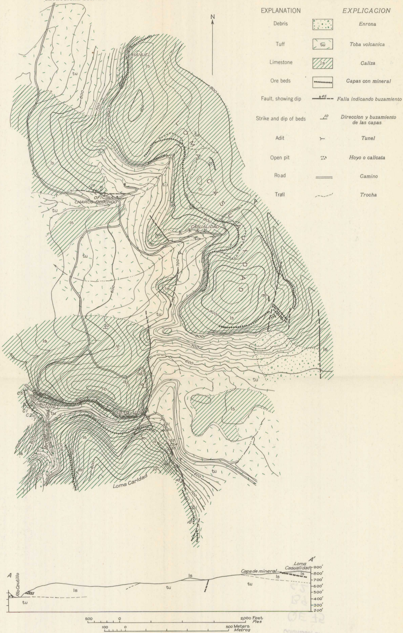
GEOLOGIC MAP AND SECTION OF PART OF CHARCO REDONDO AREA, ORIENTE PROVINCE, CUBA MAPA GEOLOGICO Y SECCION DE PARTE DEL COTO CHARCO REDONDO, PROVINCIA DE ORIENTE, CUBA
