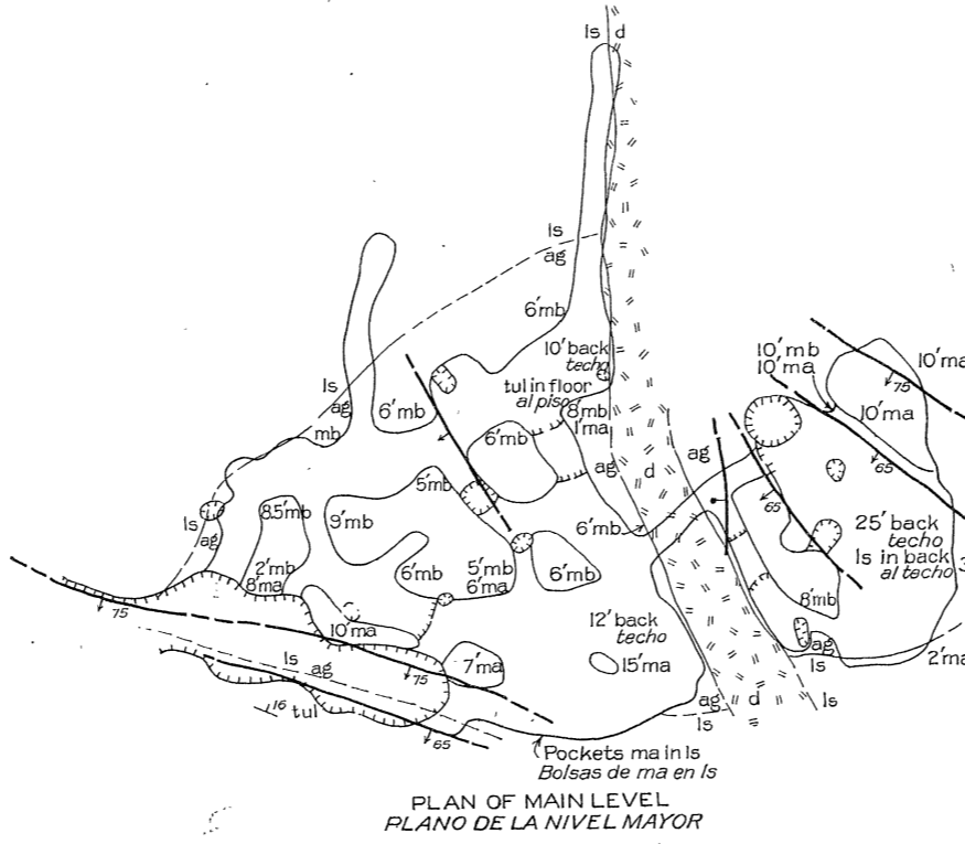
MAIN WORKINGS TRABAJOS PRINCIPALE
