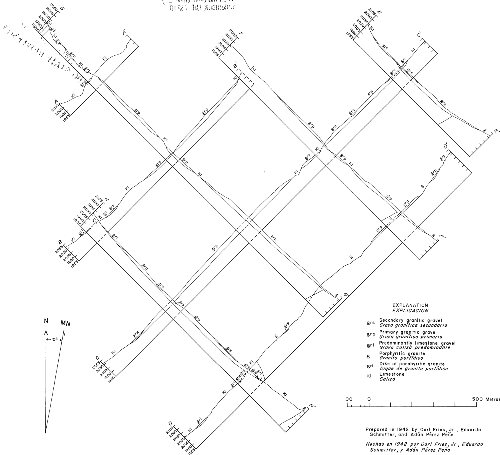
SECTIONS OF THE REALEJO BASIN, STATE OF SAN LUIS POTOSI, MEXICO SECCIONES EN LA CUENCA DE REALEJO, ESTADO DE SAN LUIS POTOSI
