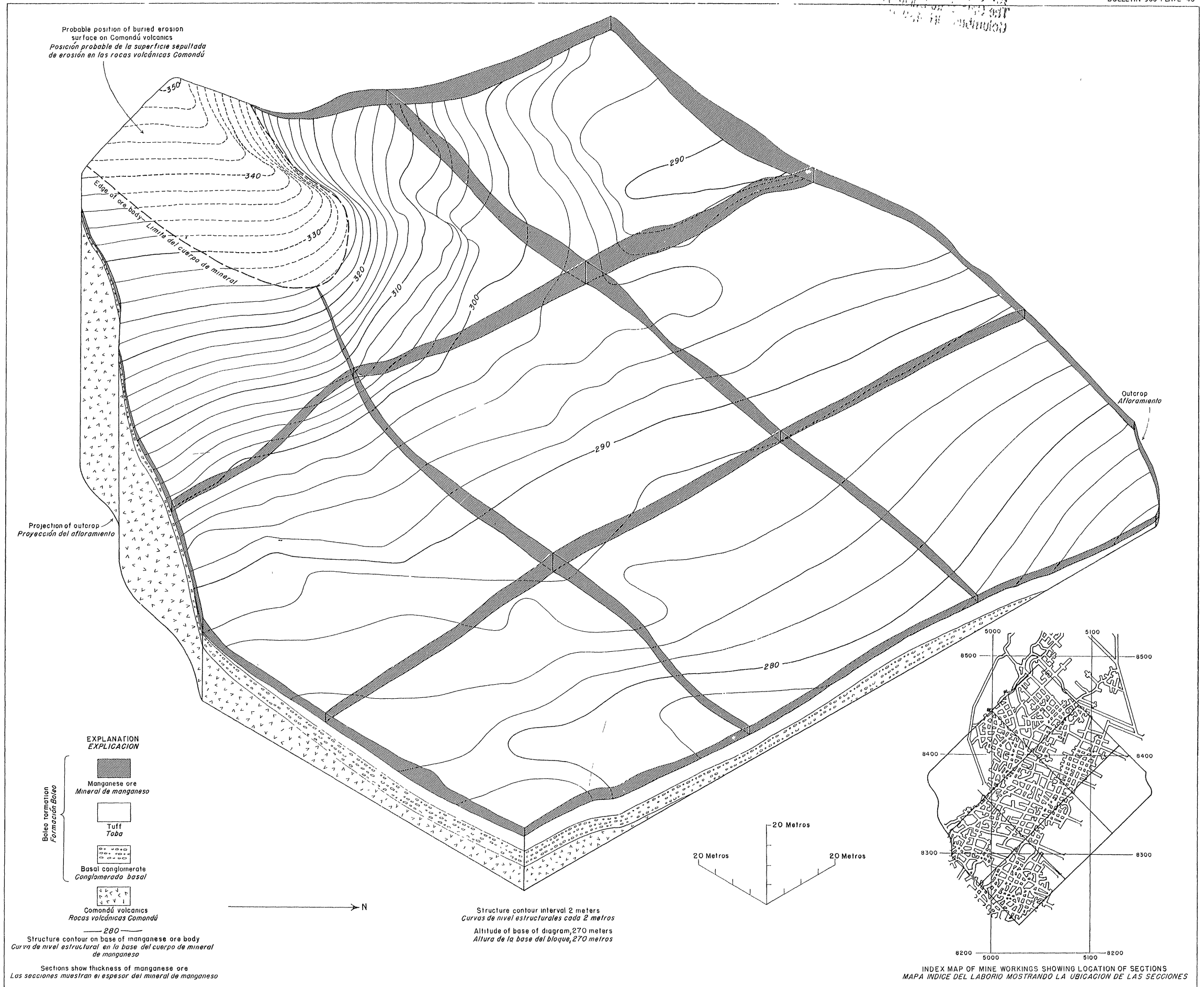
BLOCK DIAGRAM SHOWING STRUCTURE AND THICKNESS OF MANGANESE ORE, LUCIFER MINE, BAJA CALIFORNIA, MEXICO BLOQUE DIAGRAMATICO QUE MUESTRA LA ESTRUCTURA Y ESPESOR DEL MINERAL DE MANGANESO, MINA LUCIFER, BAJA CALIFORNIA
