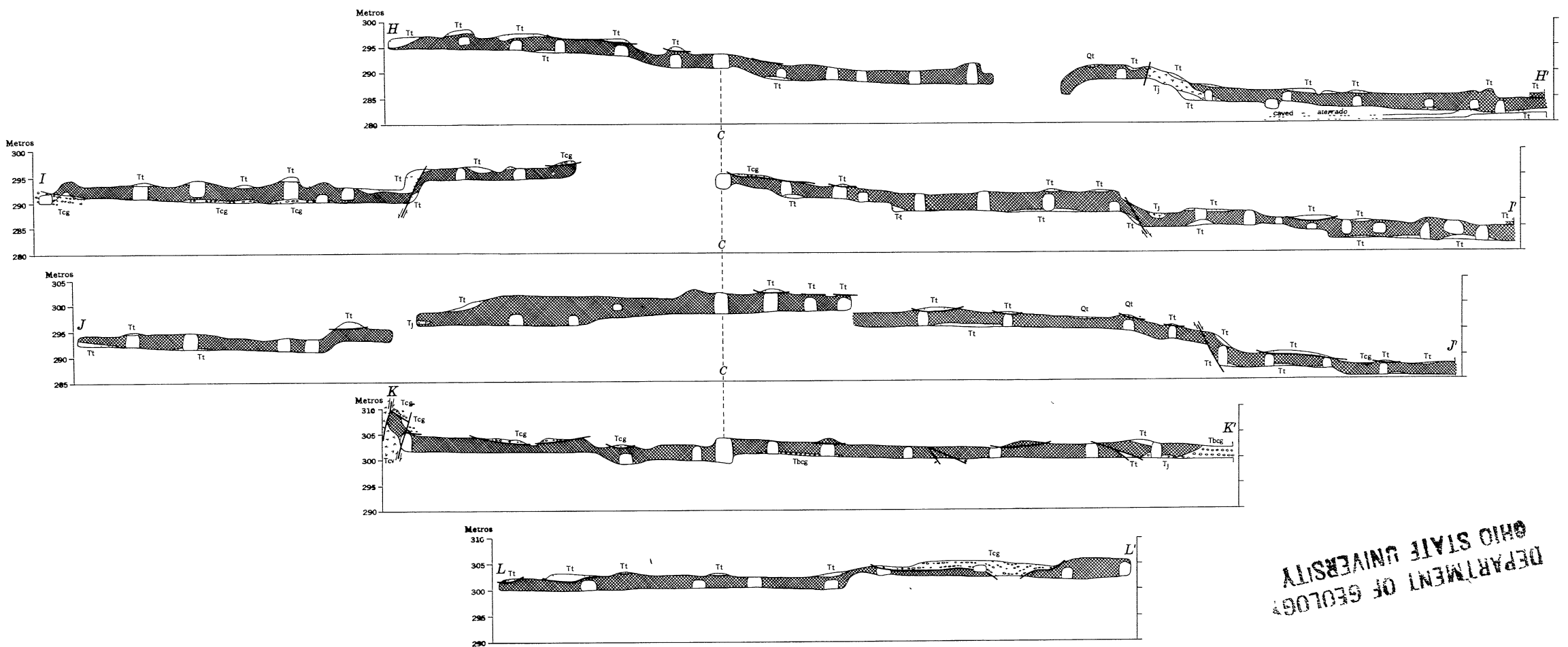
GEOLOGIC SECTIONS ALONG PRINCIPAL UNDERGROUND WORKINGS, LUCIFER MANGANESE MINE, BAJA CALIFORNIA, MEXICO SECCIONES GEOLOGICAS A LO LARGO DE LAS LABORES PRINCIPALES DE LA MINA DE MANGANESO LUCIFER, BAJA CALIFORNIA
