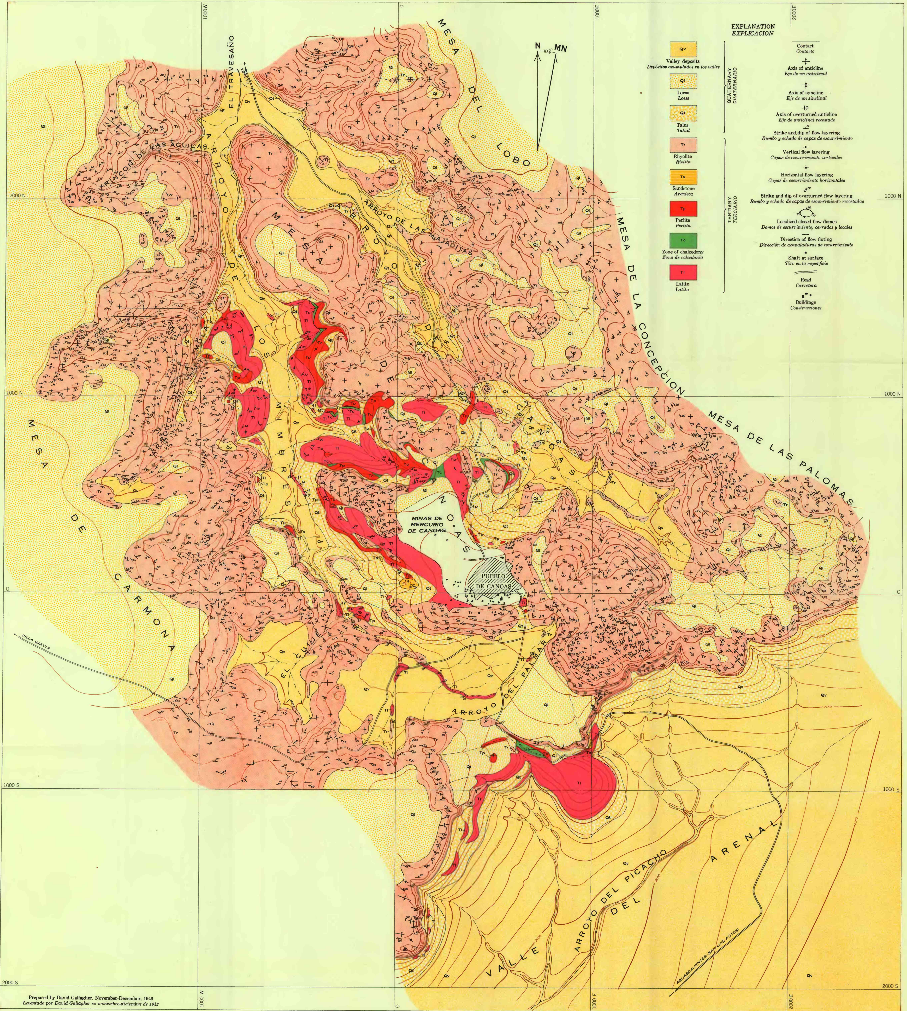
GEOLOGIC MAP OF THE CANOAS QUICKSILVER DISTRICT, STATE OF ZACATECAS, MEXICO PLANO GEOLOGICO DE LA ZONA MERCURIO DE CANOAS, ESTADO DE ZACATECAS
