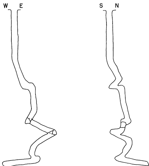
PLAN AND PROJECTION OF POZO 122 PLANO Y PROYECCION DE POZO 122
