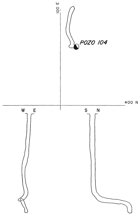
PLAN AND PROJECTION OF POZO 104 PLANO Y PROYECCION DE POZO 104
