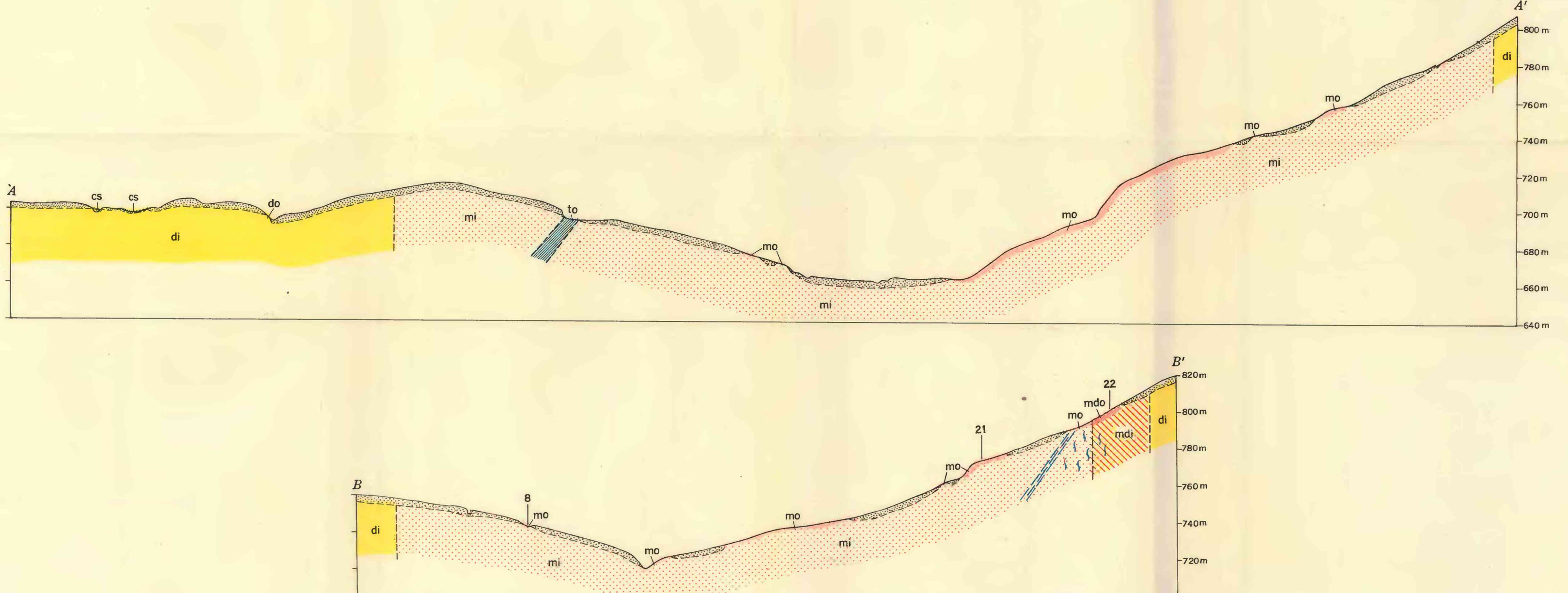
GEOLOGIC MAP AND SECTIONS OF THE PEDRA PRETA MAGNESITE DEPOSIT, SERRA DAS ÉGUAS, BRUMADO, BAHIA, BRAZIL MAPA GEOLÓGICO E SECÇÕES DO DEPÓSITO DE MAGNESITA DE PEDRA PRETA DA SERRA DAS ÉGUAS, BRUMADO, BAHIA, BRASIL
