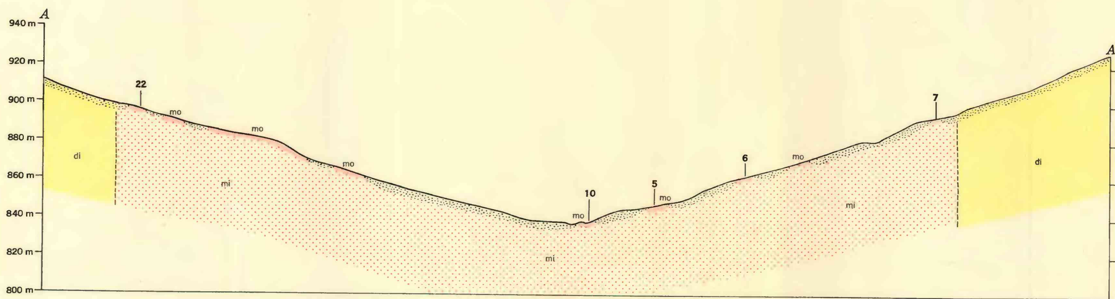
GEOLOGIC MAP AND SECTION OF THE CATIBOABA MAGNESITE DEPOSIT, BRUMADO, BAHIA, BRAZIL MAPA GEOLÓGICO E SEÇÃO DO DEPÓSITO DE MAGNESITA DE CATIBOABA, BRUMADO, BAHIA, BRASIL
