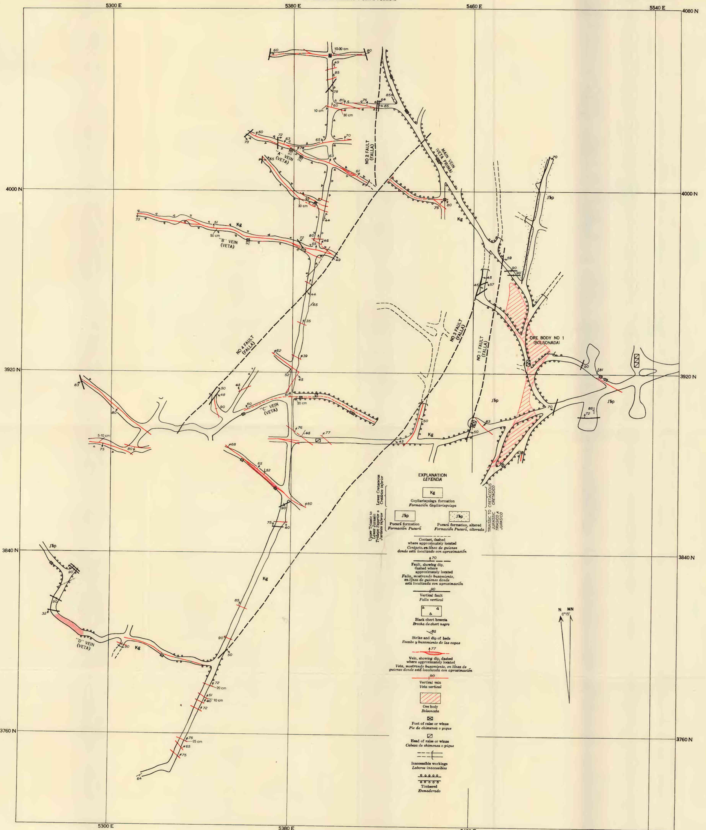
MAP OF THE 3900 LEVEL, ATACOCHA MINE, DEPARTAMENTO DE PASCO, PERU MAPA DEL NIVEL 3900, MINA ATACOCHA, DEPARTAMENTO DE PASCO, PERU
