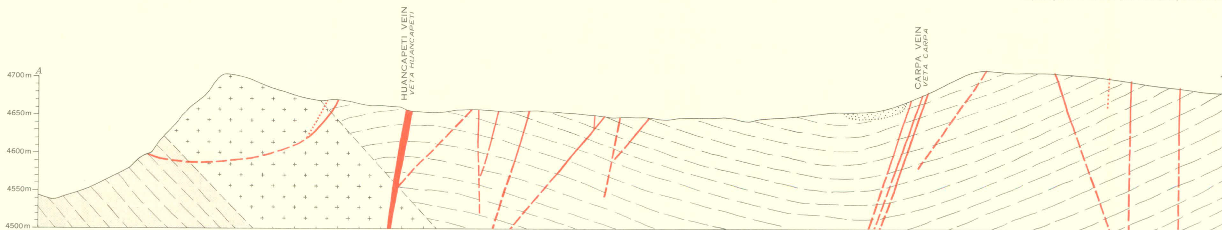
GEOLOGIC MAP AND SECTION OF THE HUANCAPETI DEPOSIT, PERU MAPA Y PERFIL GEOLOGICO DEL DEPOSITO HUANCAPETI, PERU
