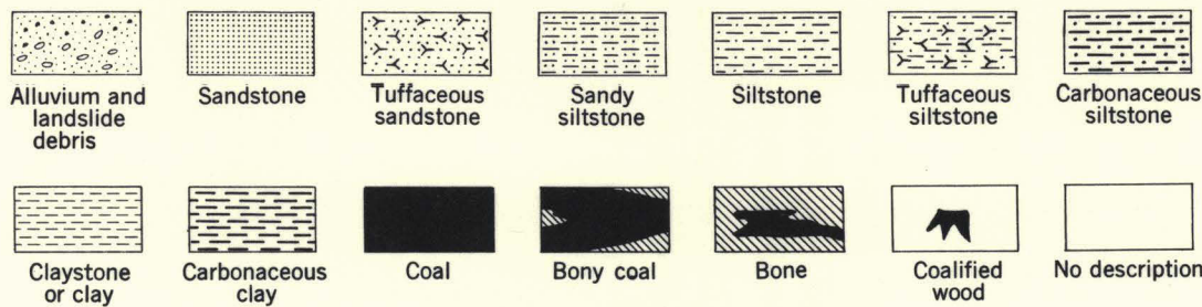
SECTIONS OF COAL BEDS IN T. 11 N., R. 2 W.; T. 10 N., R. 2 W.; T. 10 N., R. 1 W.; T. 10 N., R. 1 E., T. 9 N., R. 2 W.; AND T. 9 N., R. 1 W., LEWIS AND COWLITZ COUNTIES, WASHINGTON
