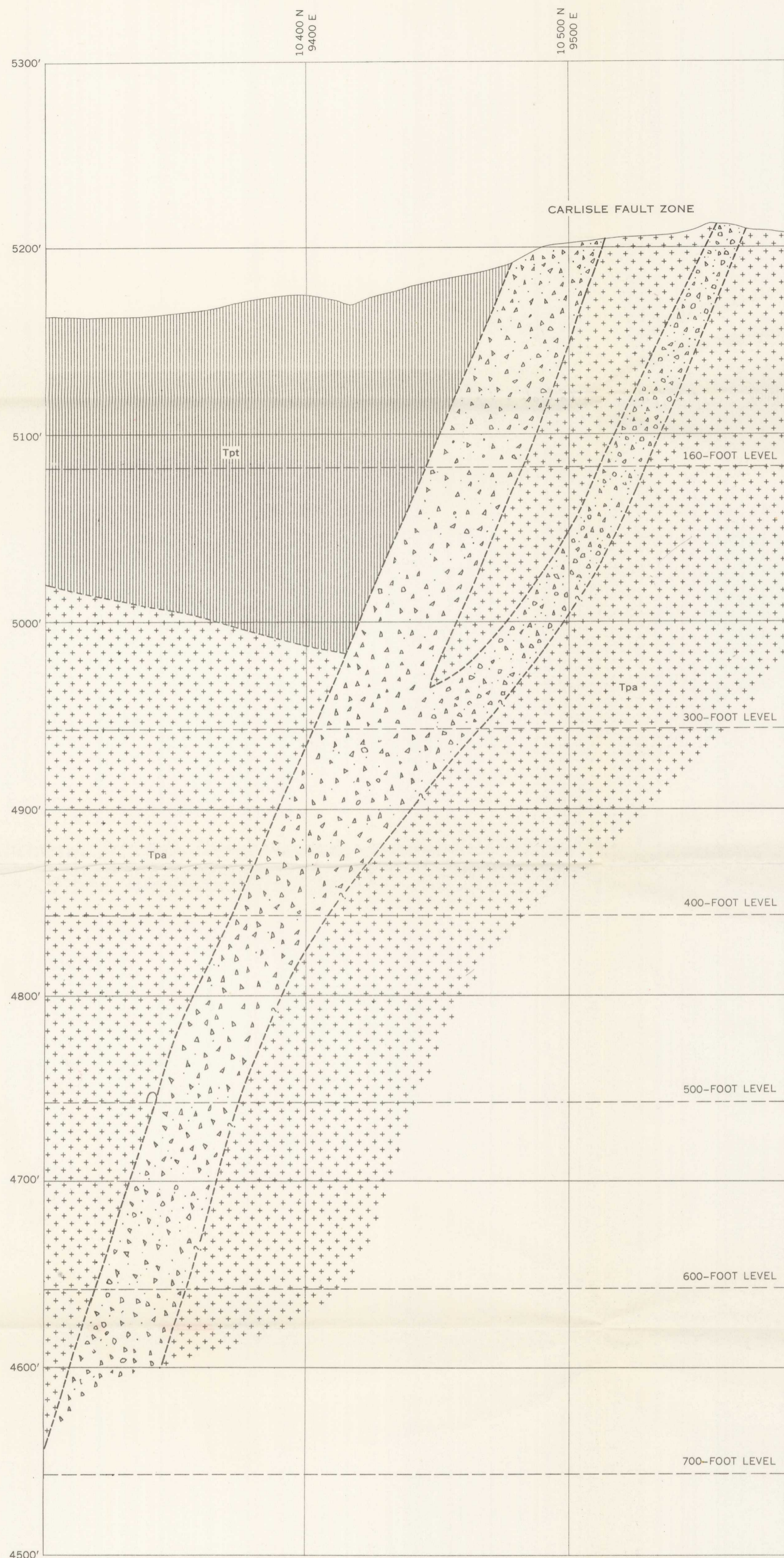
SECTION A-A'
