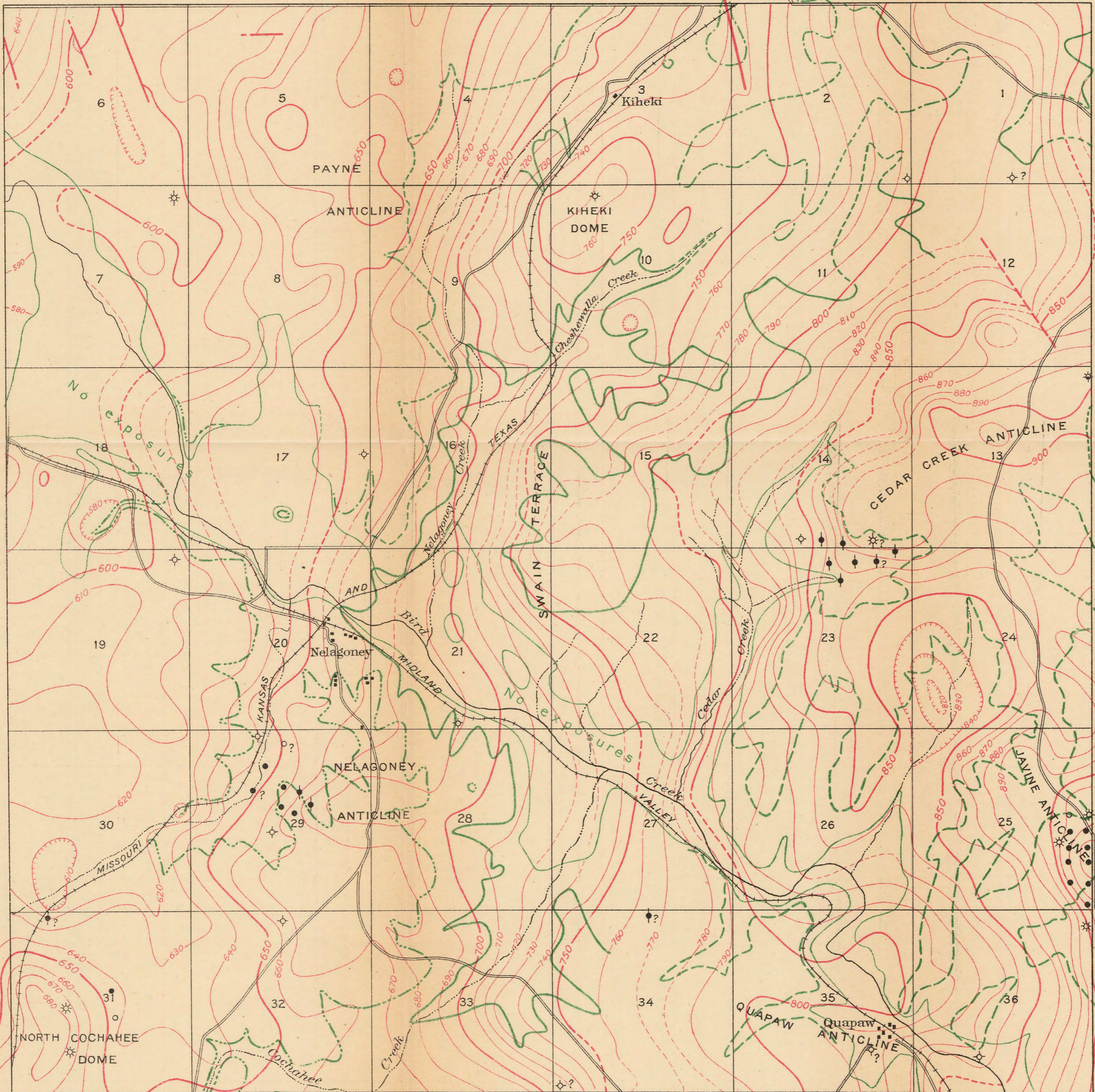
MAP SHOWING GEOLOGIC STRUCTURE OF T. 25 N., R. 10 E.
