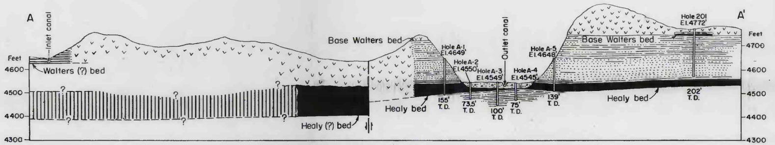
Section A-A'
