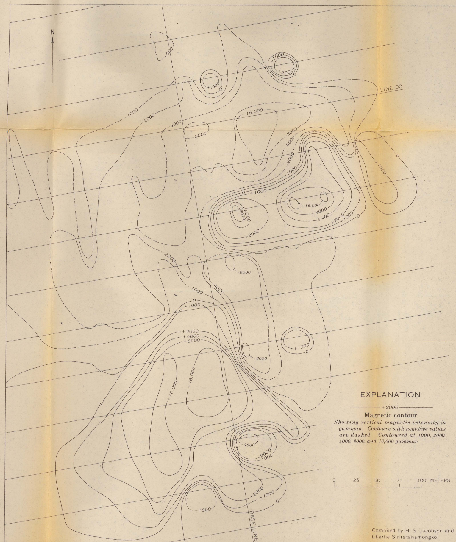
B. MAGNETIC MAP
