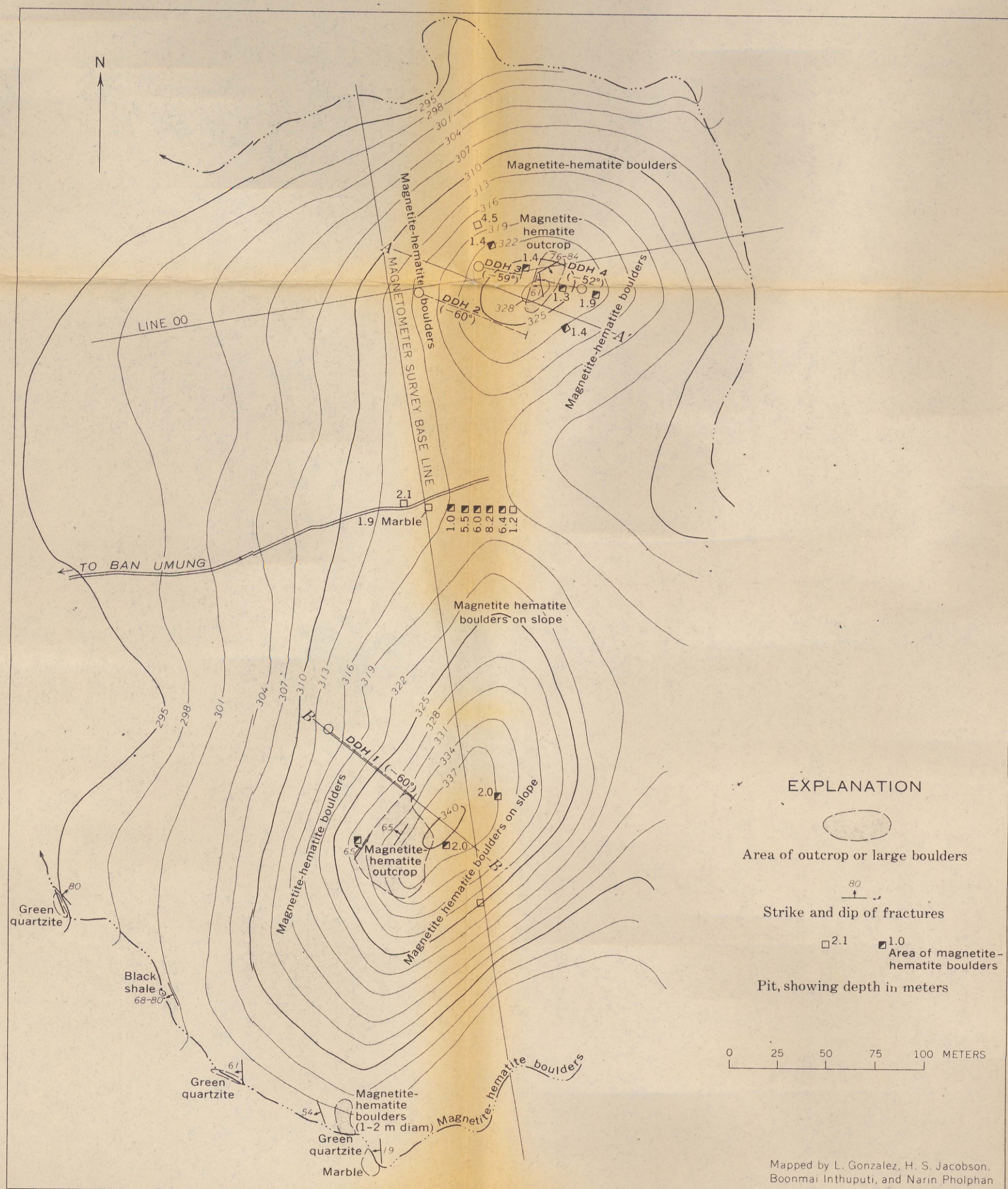
A. GEOLOGIC MAP
