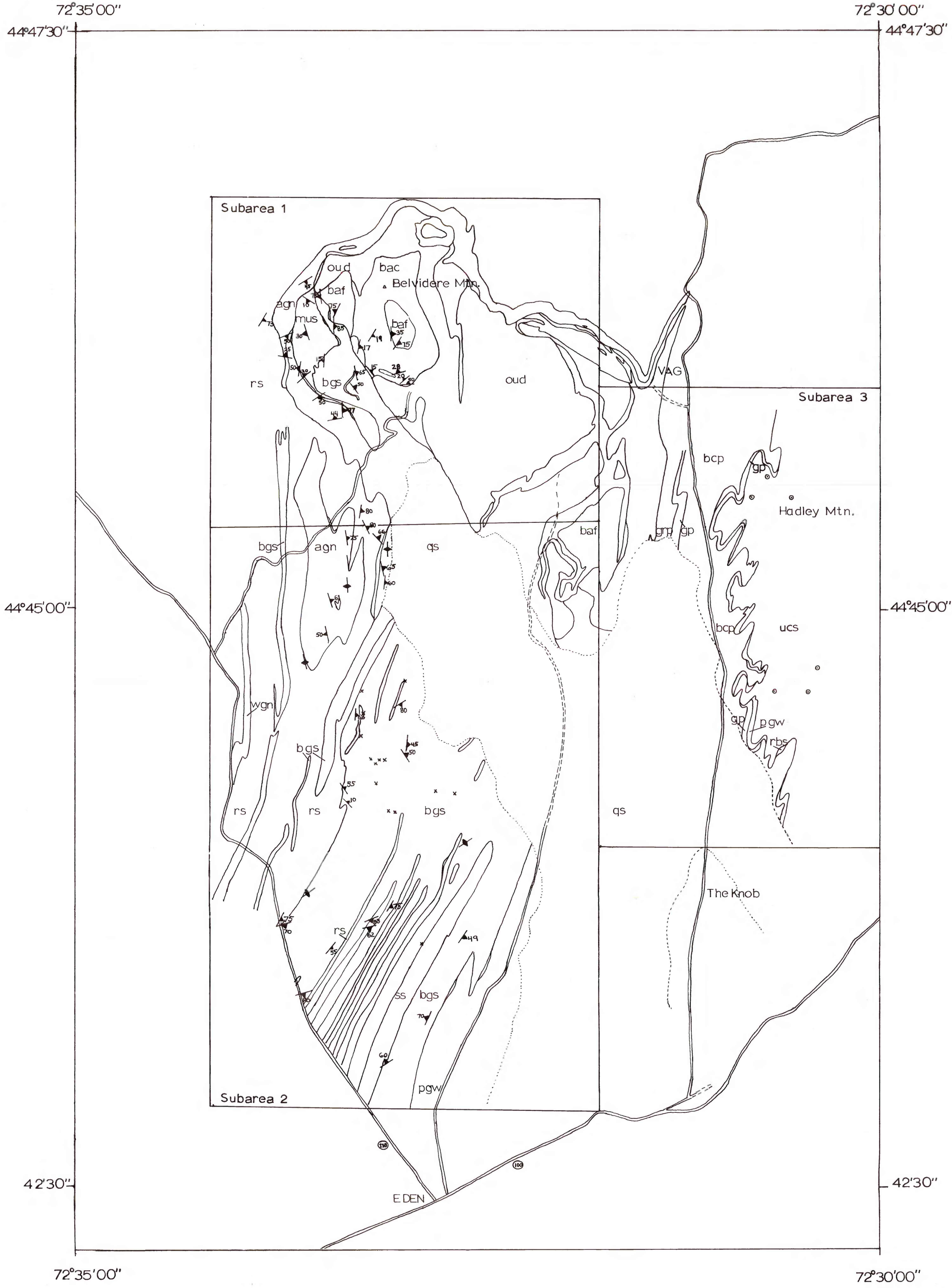
PLATE III F1 STRUCTURE MAP
