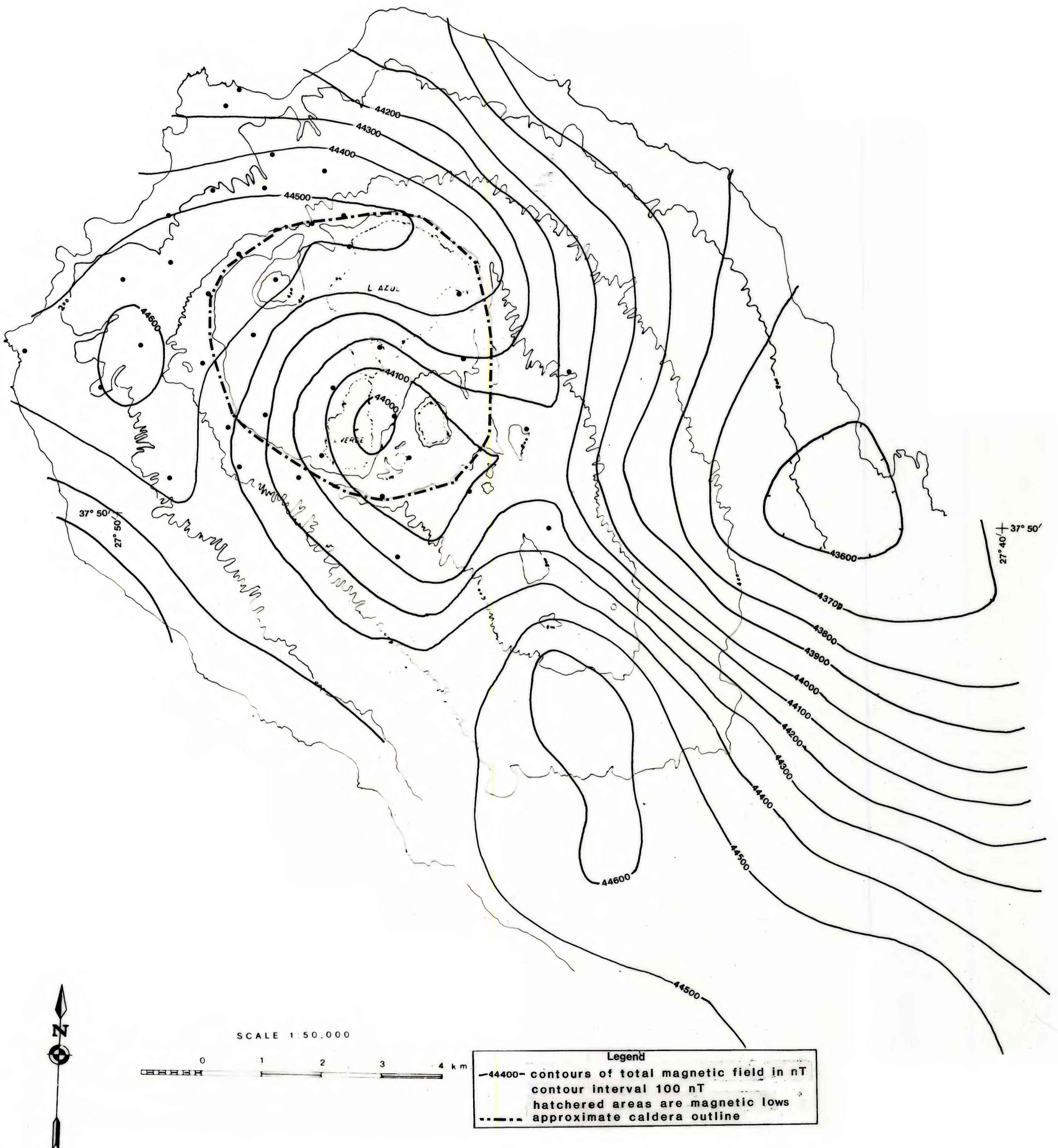
Plate 8. Total field aeromagnetic map of the Sete Cidades area, São Miguel Island, Azores
