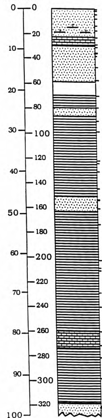
Fig. III-4. Core log, Borehole D
