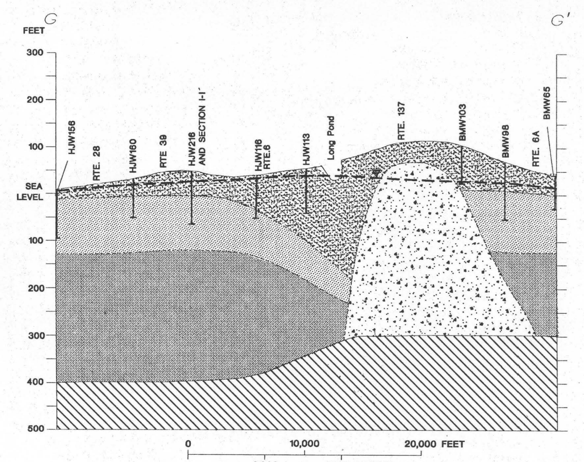
G. Hydrogeologic section G-G'
