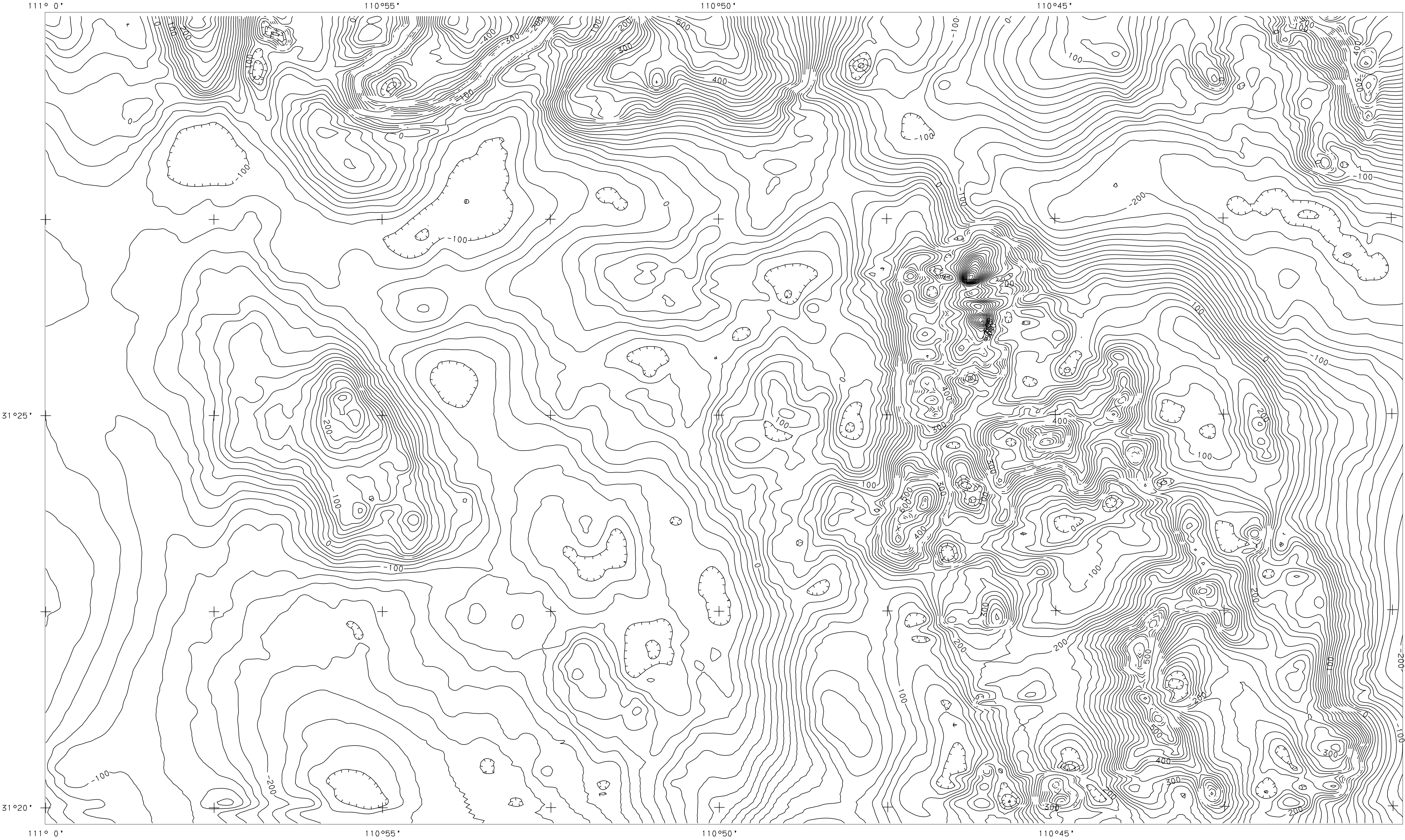
Simons map aeromag anomaly
