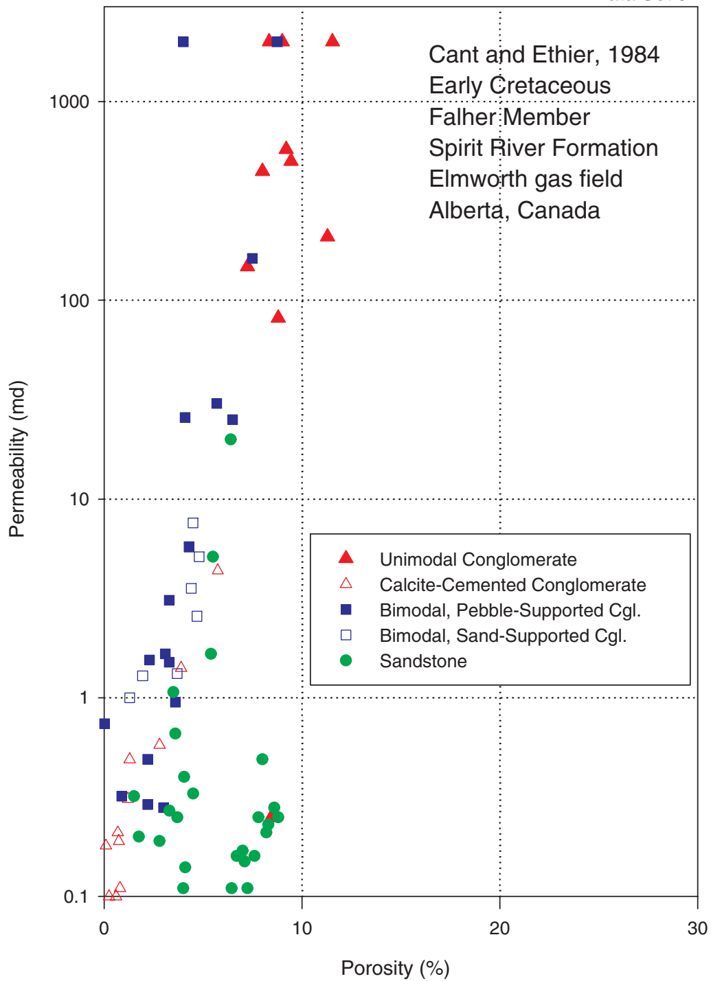
Data Set 9
