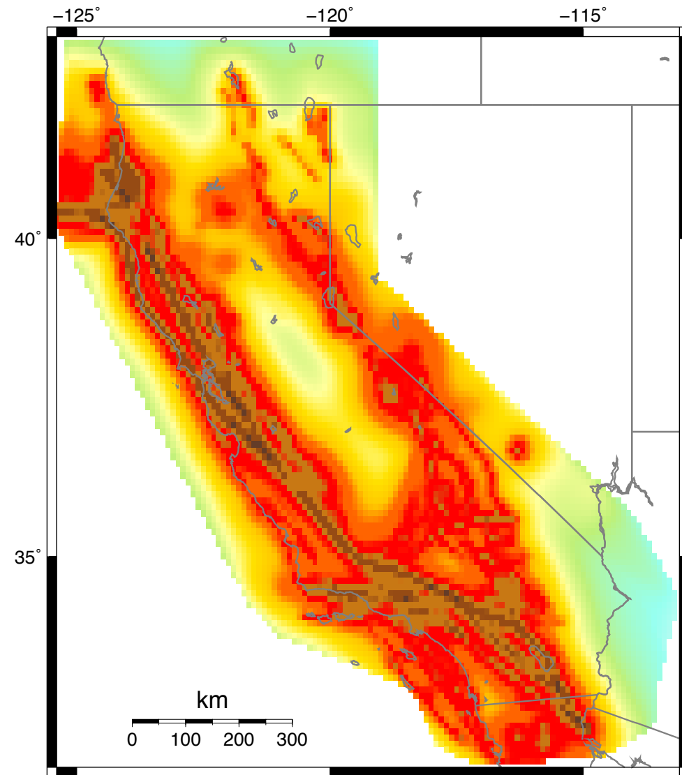
UCERF 3.3
