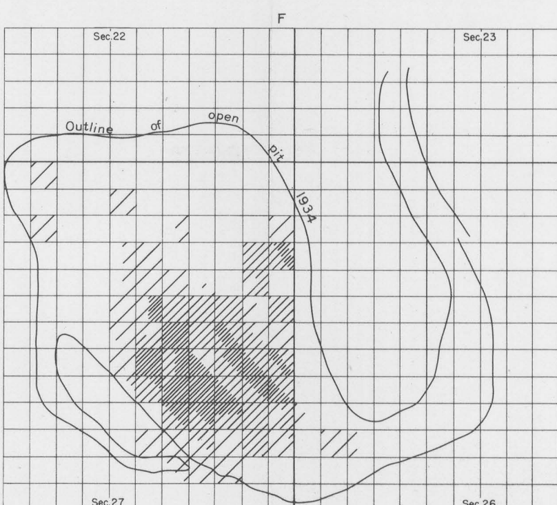
PEGMATITE
