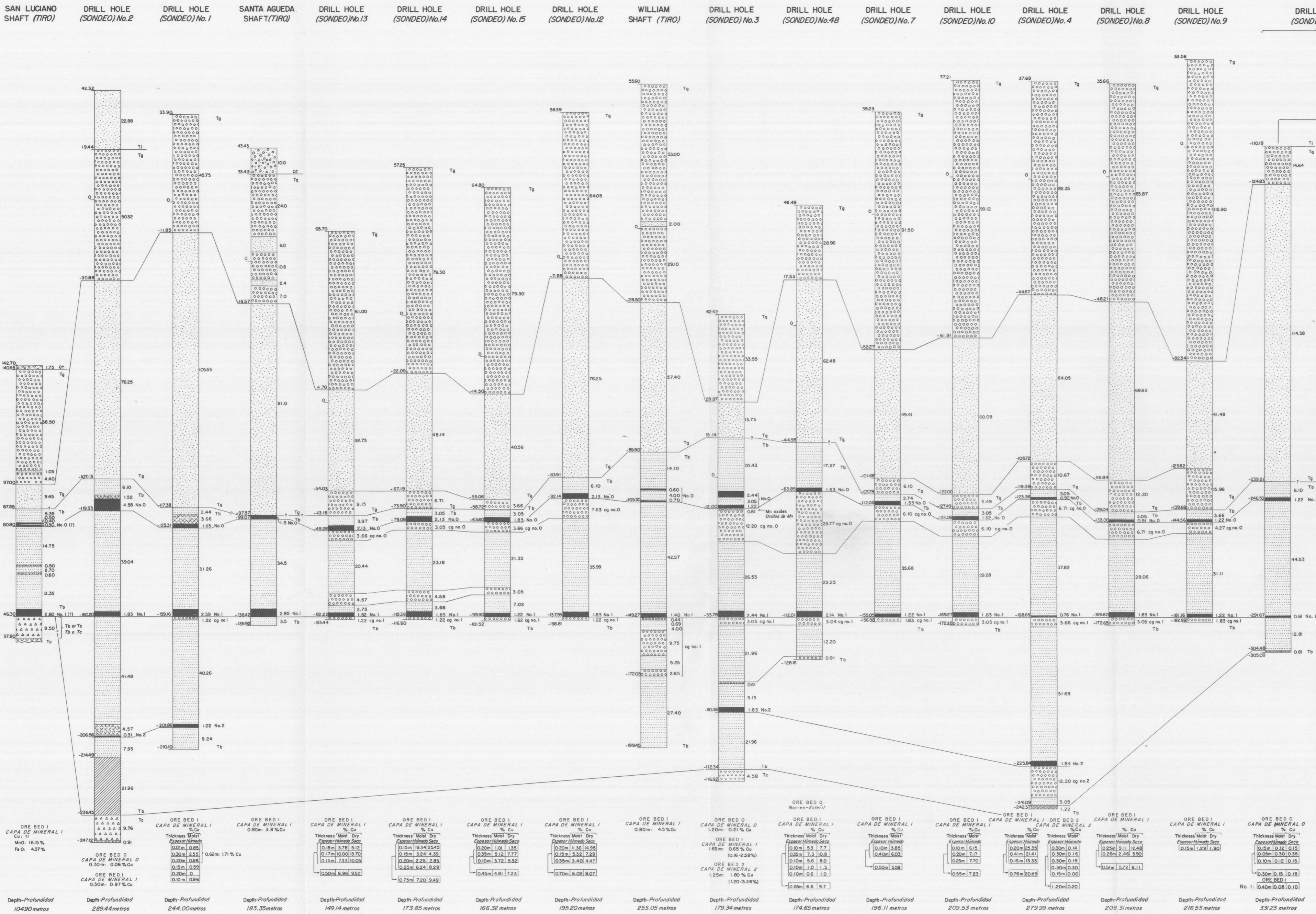
COLUMNAR SECTIONS OF SHAFTS AND DRILL HOLES IN THE BOLEO COPPER DISTRICT: AREA IN ARROYO DE SANTA AGUEDA AND VICINITY (NORTHERN GROUP) SECCIONES COLUMNARES DE LOS TIROS Y SONDEOS EN EL DISTRITO CUPRIFERO DE BOLEO: AREA EN EL ARROYO DE SANTA AGUEDA Y SU VEGINDAD (GRUPO NORTE)
