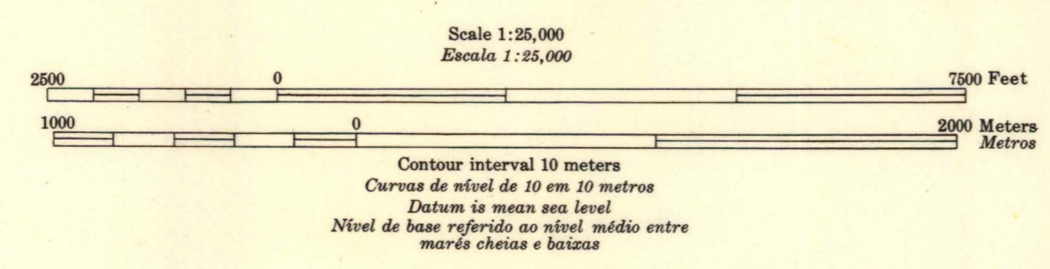
GEOLOGIC MAP AND SECTION OF THE CONGONHAS QUADRANGLE, MINAS GERAIS, BRAZIL. MAPA GEOLÓGICO E PERFIL DO QUADRÂNGULO DE CONGONHAS, MINAS GERAIS, BRASIL
