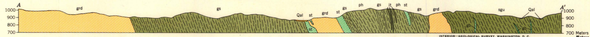
GEOLOGIC MAP AND SECTION OF THE CONGONHAS QUADRANGLE, MINAS GERAIS, BRAZIL. MAPA GEOLÓGICO E PERFIL DO QUADRÂNGULO DE CONGONHAS, MINAS GERAIS, BRASIL
