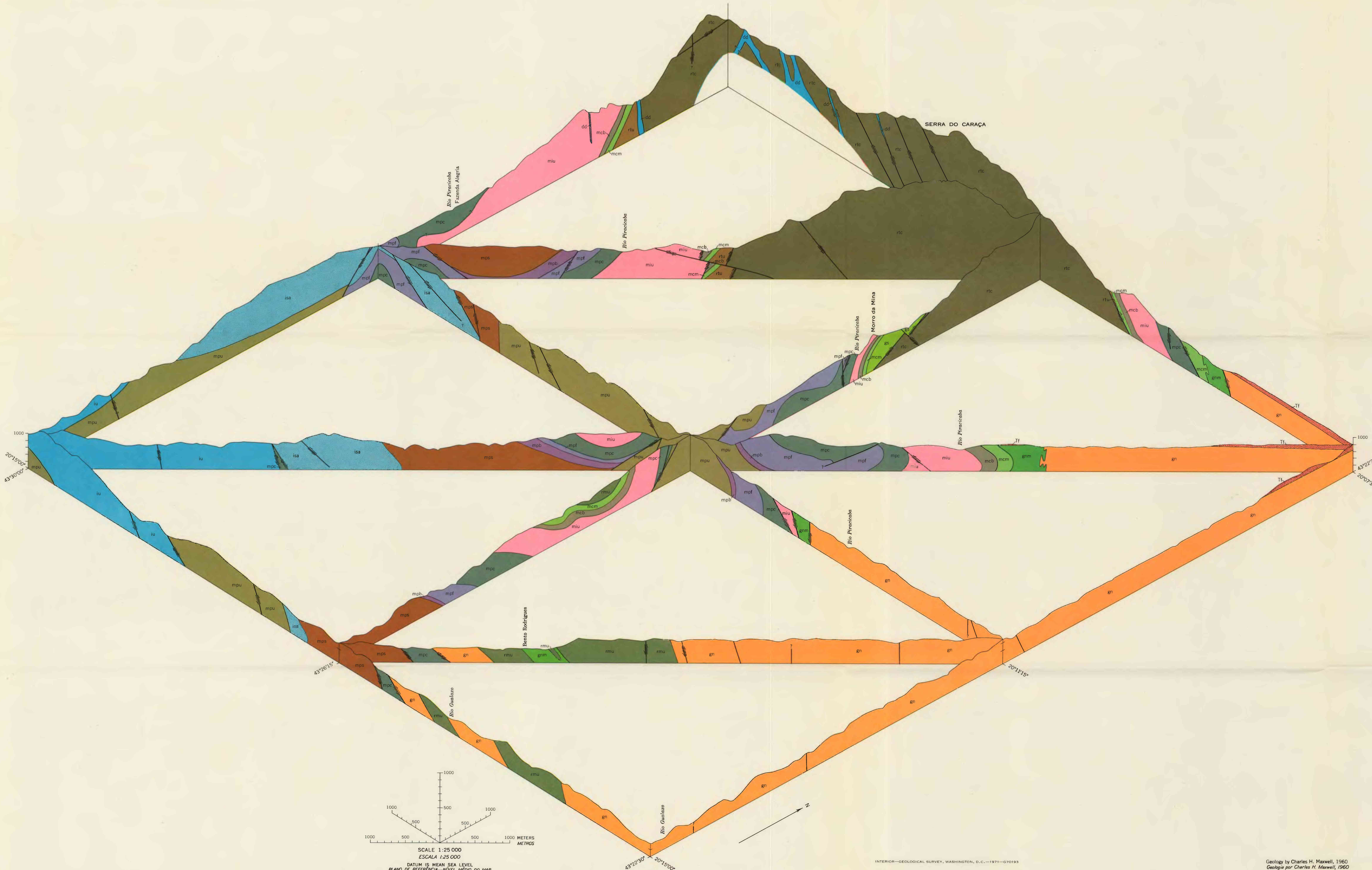
ISOMETRIC FENCE DIAGRAM AND CROSS SECTIONS OF THE SANTA RITA DURÃO QUADRANGLE, MINAS GERAIS, BRAZIL DIAGRAMA ISOMÉTRICO E SEÇÕES TRANSVERSAIS DA QUADRÍCULA DE SANTA RITA DURÃO, MINAS GERAIS, BRASIL
