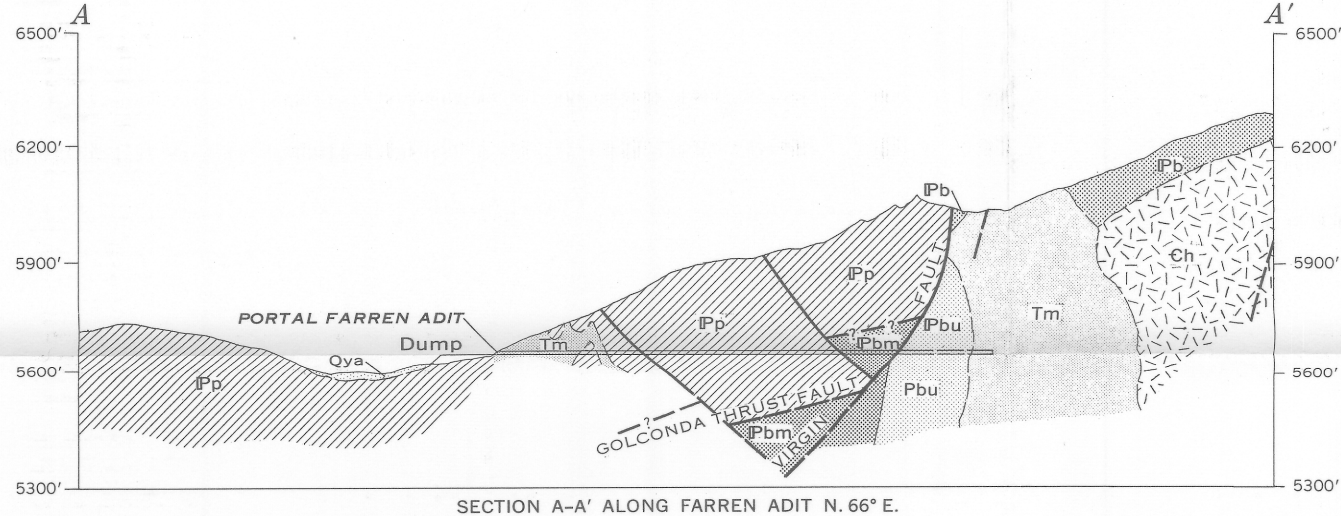
SECTION A-A' ALONG FARREN ADIT N. 66° E.
