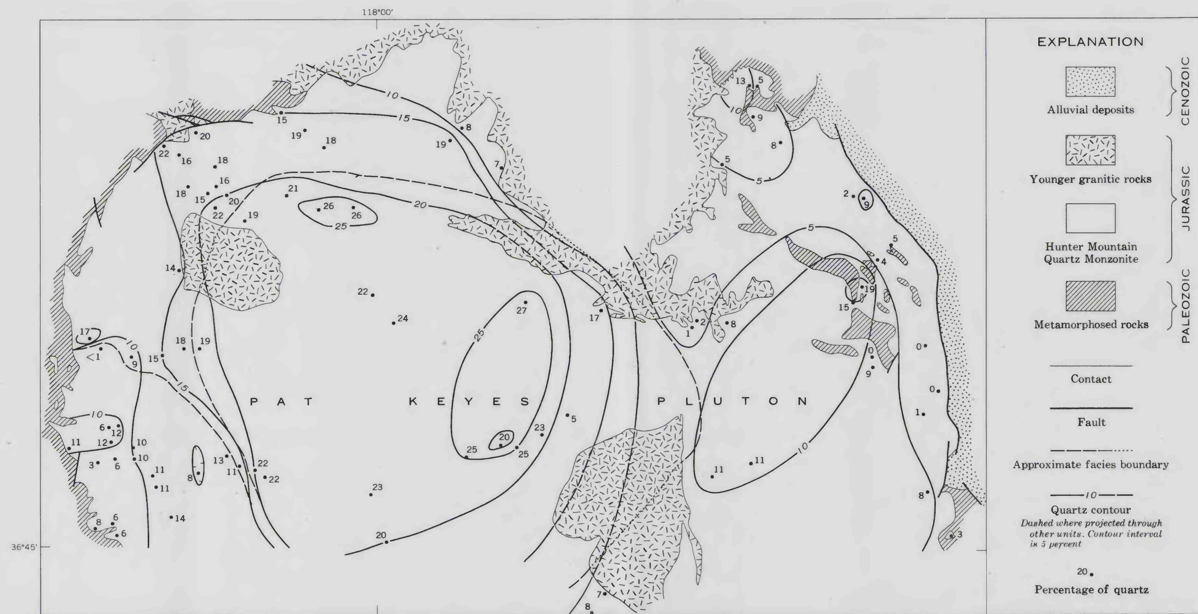
E. QUARTZ
