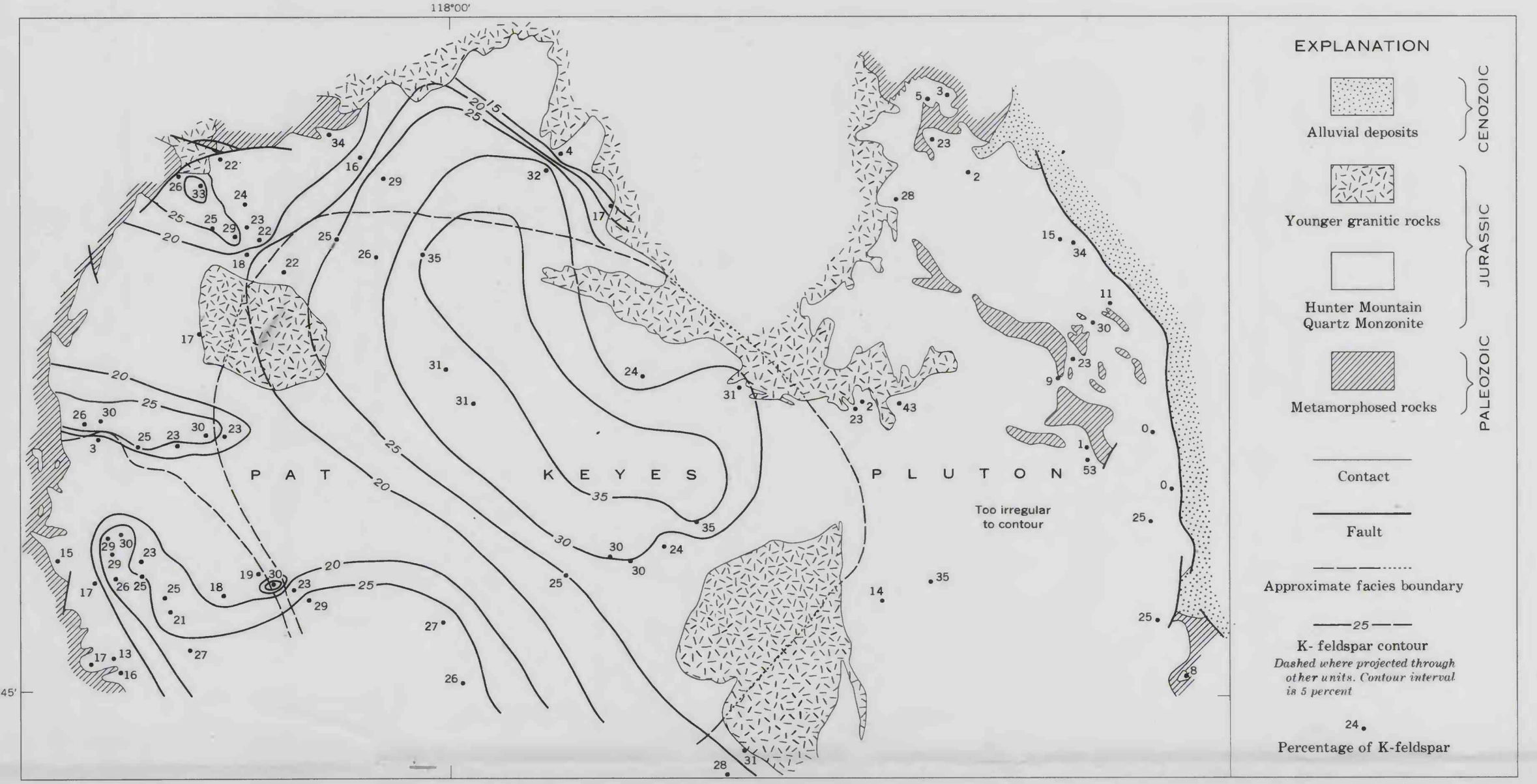
B. K-FELDSPAR
