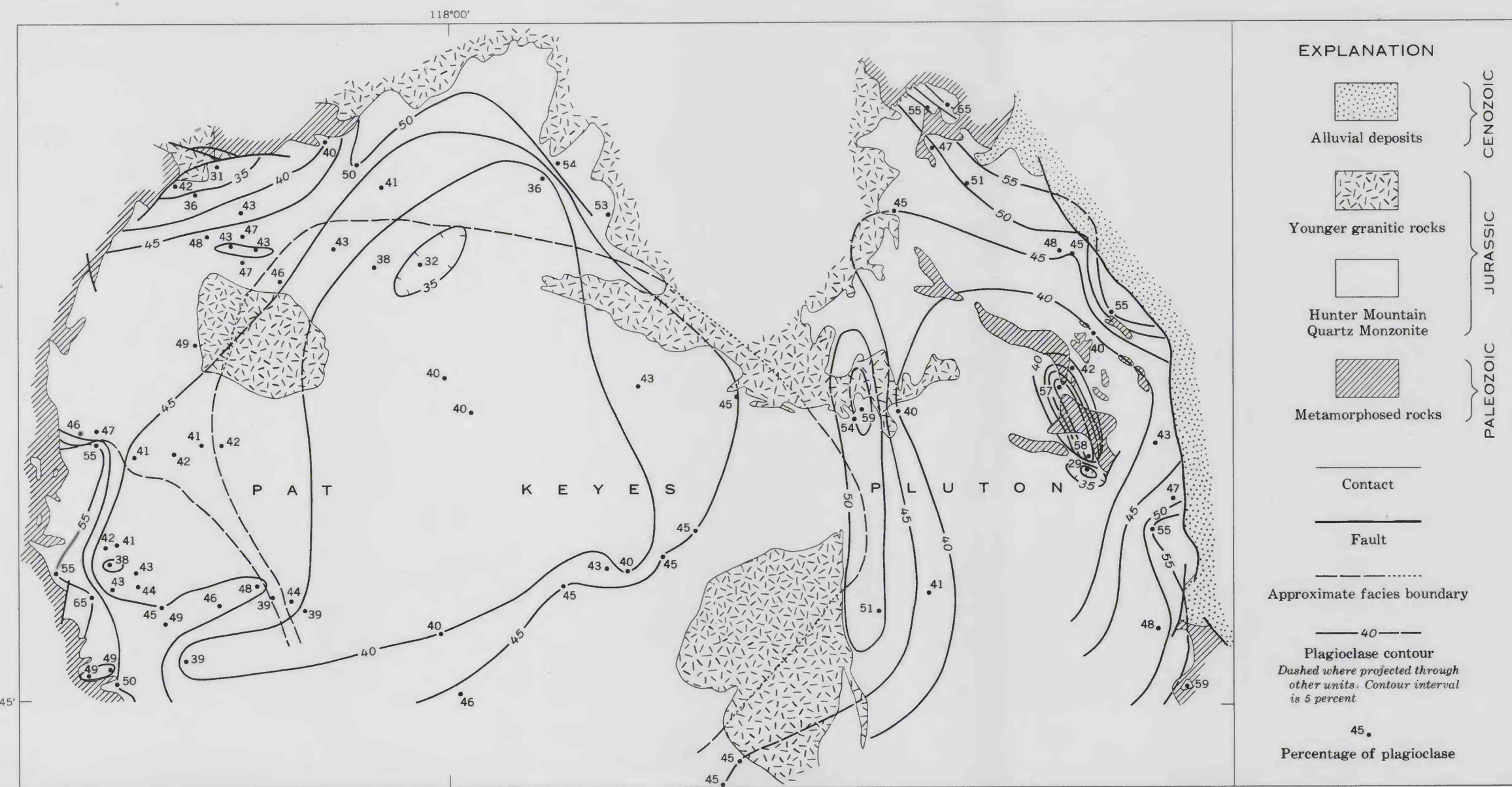
C. PLAGIOCLASE
