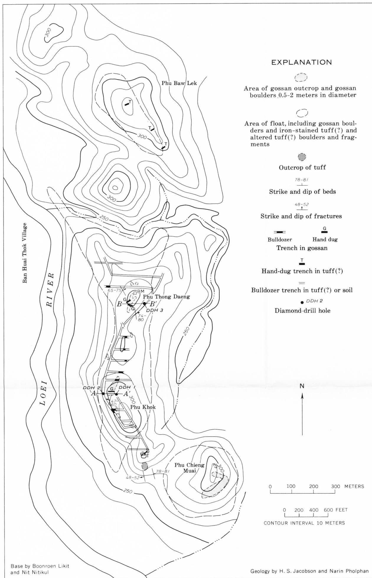
A. GEOLOGIC MAP
