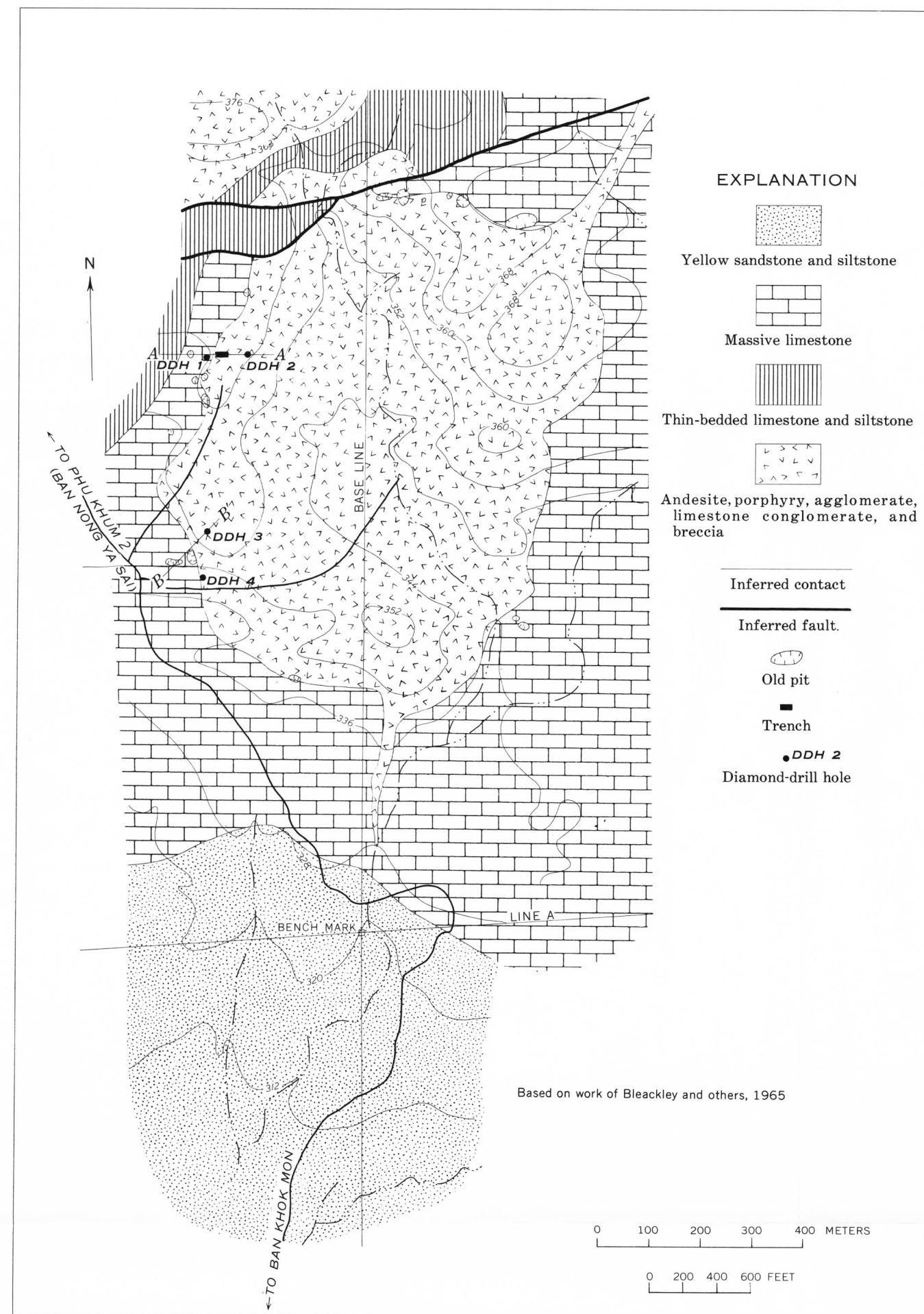
A. GEOLOGIC MAP
