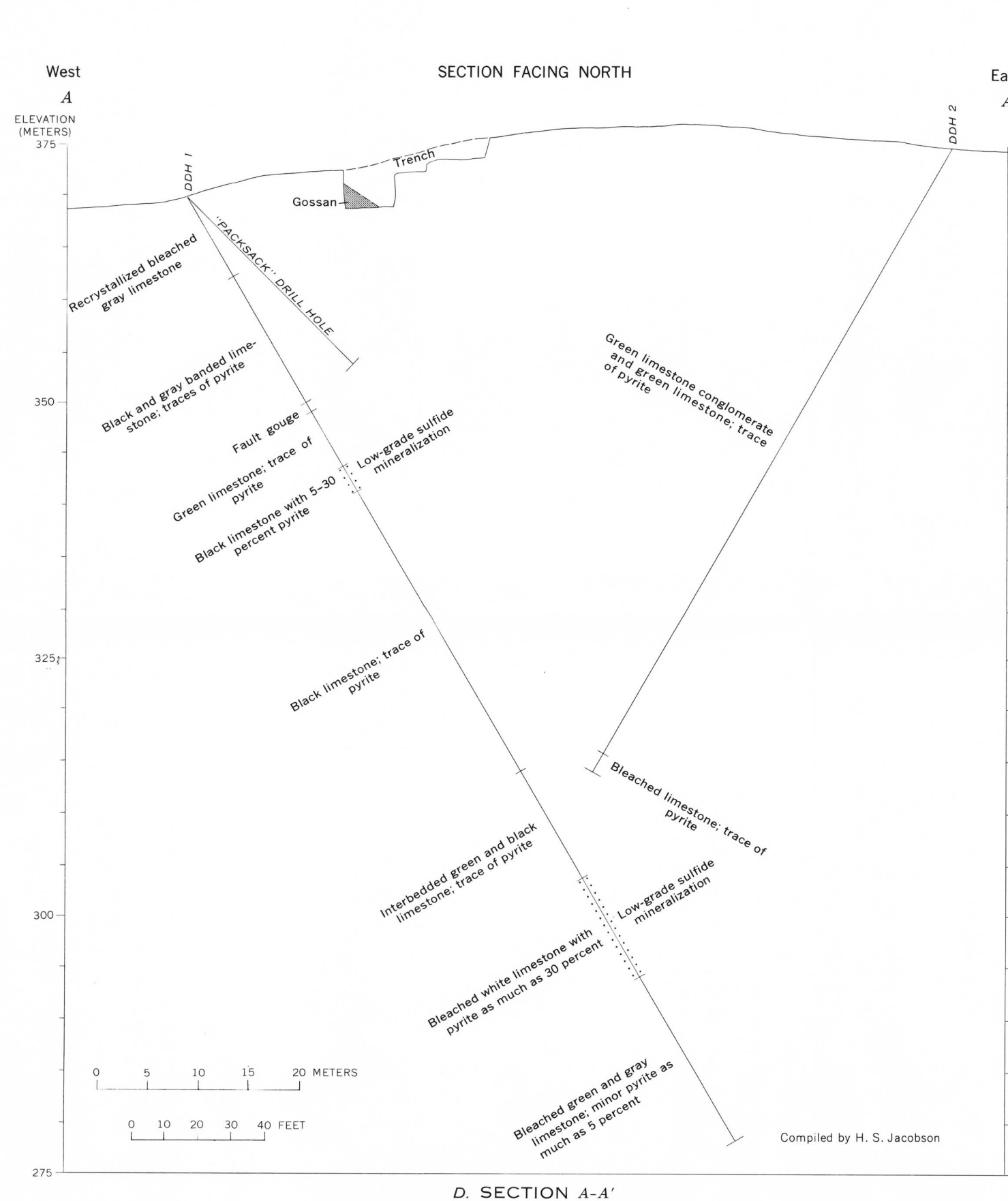
D. SECTION A-A'
