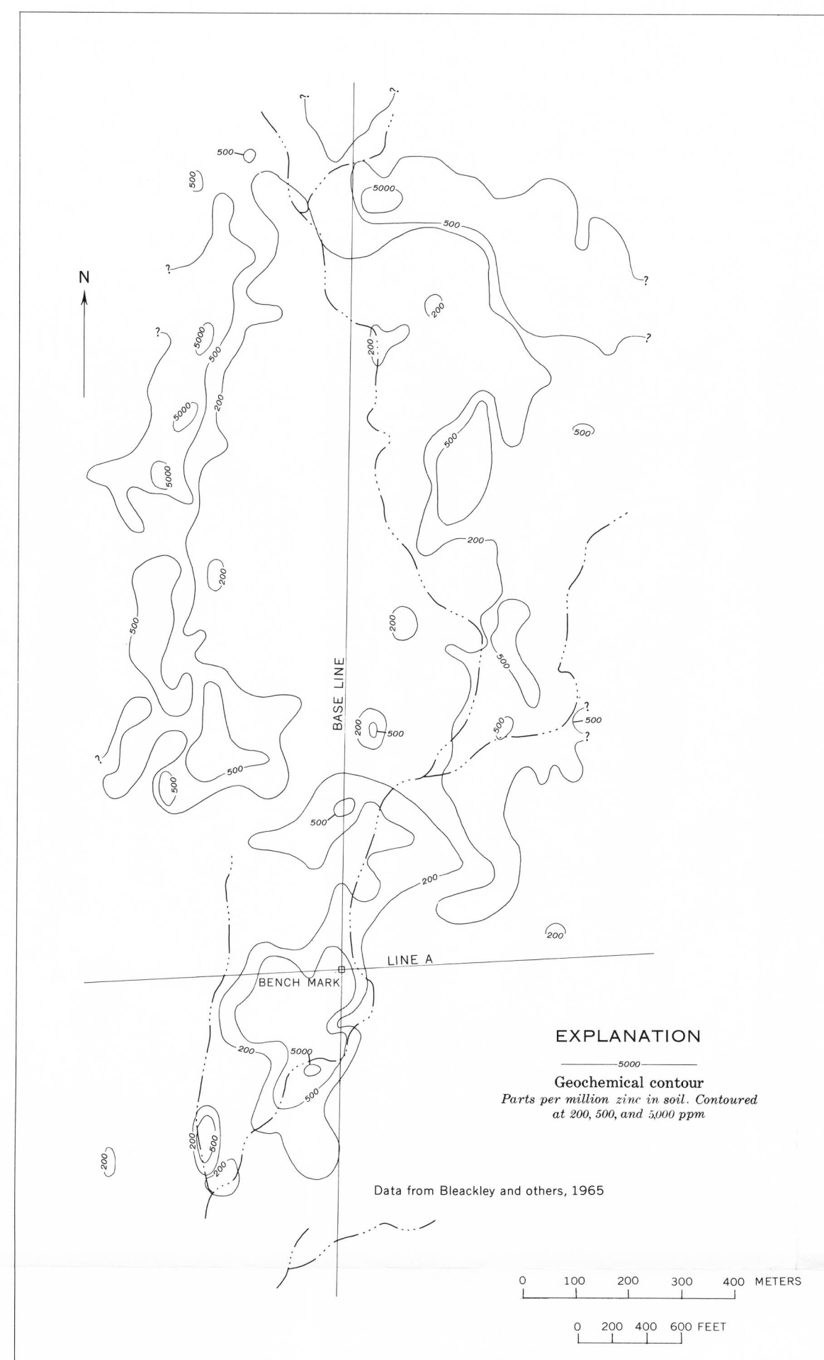
B. GEOCHEMICAL MAP (ZINC)
