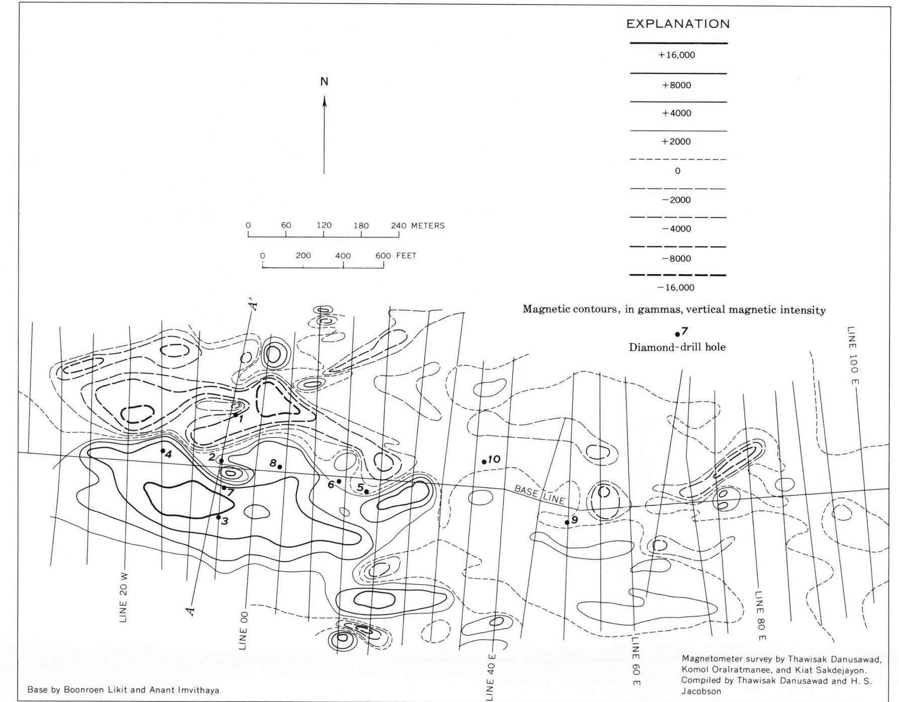
B. MAGNETIC MAP
