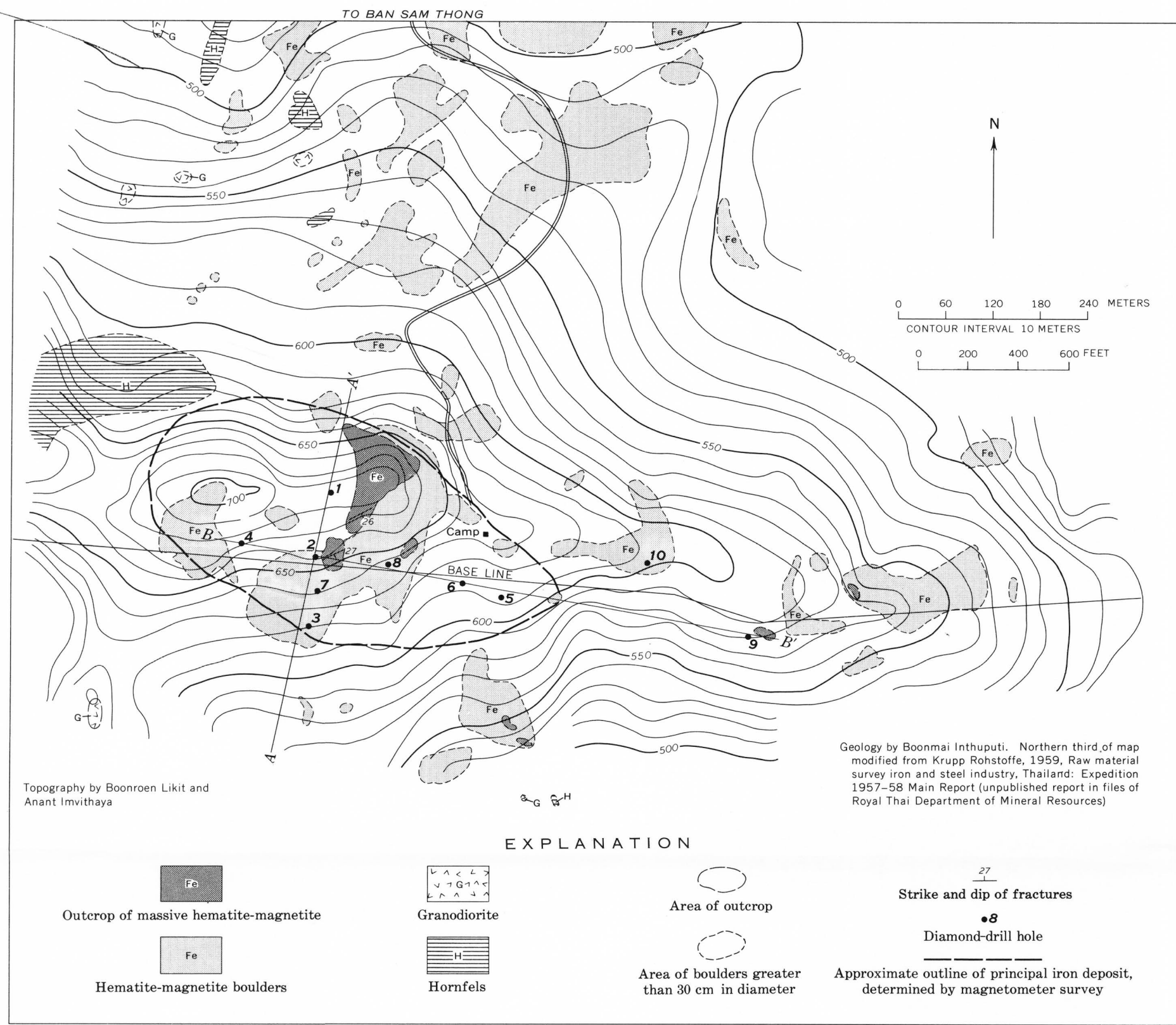
A. GEOLOGIC MAP
