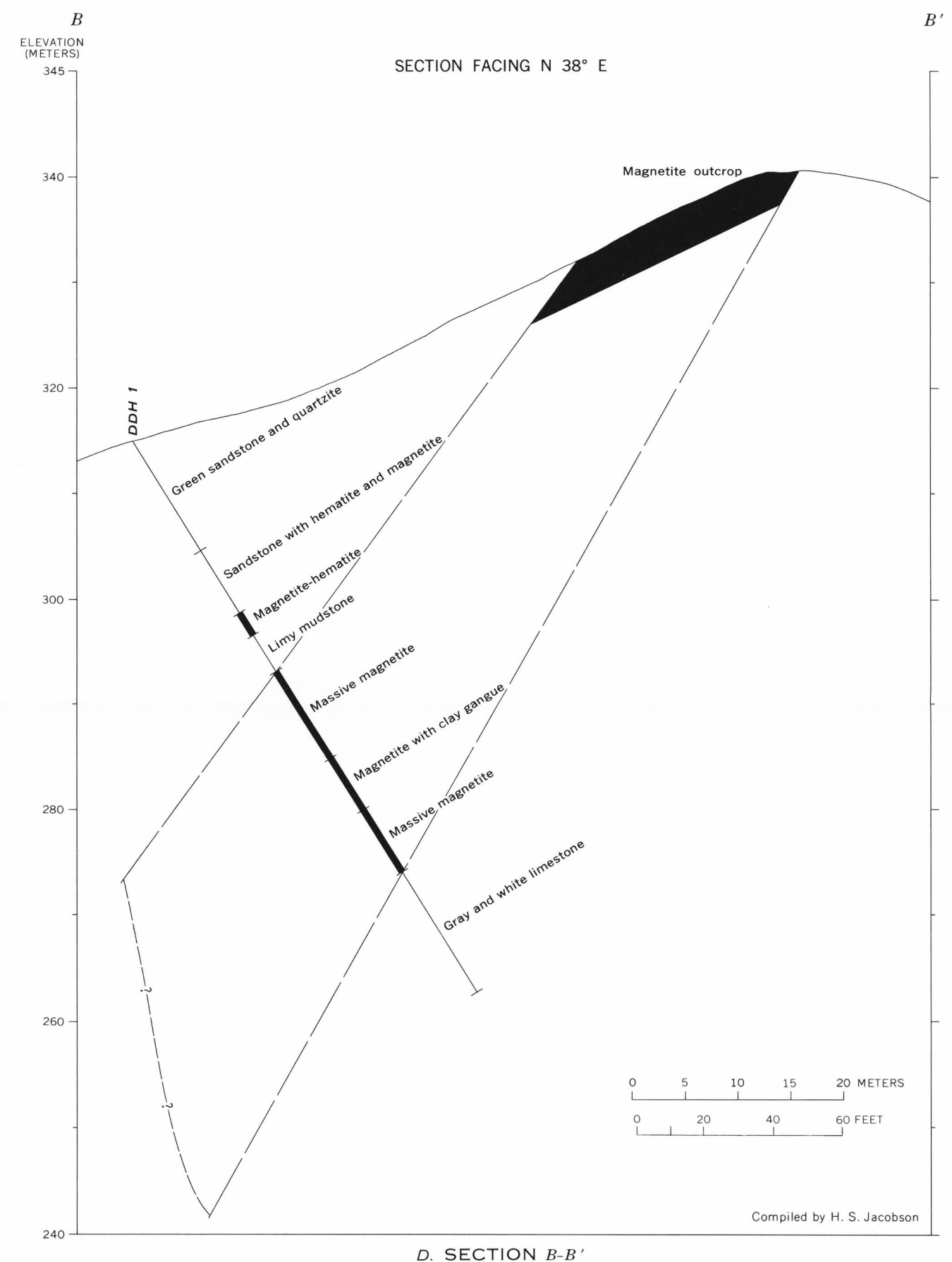
D. SECTION B-B'
