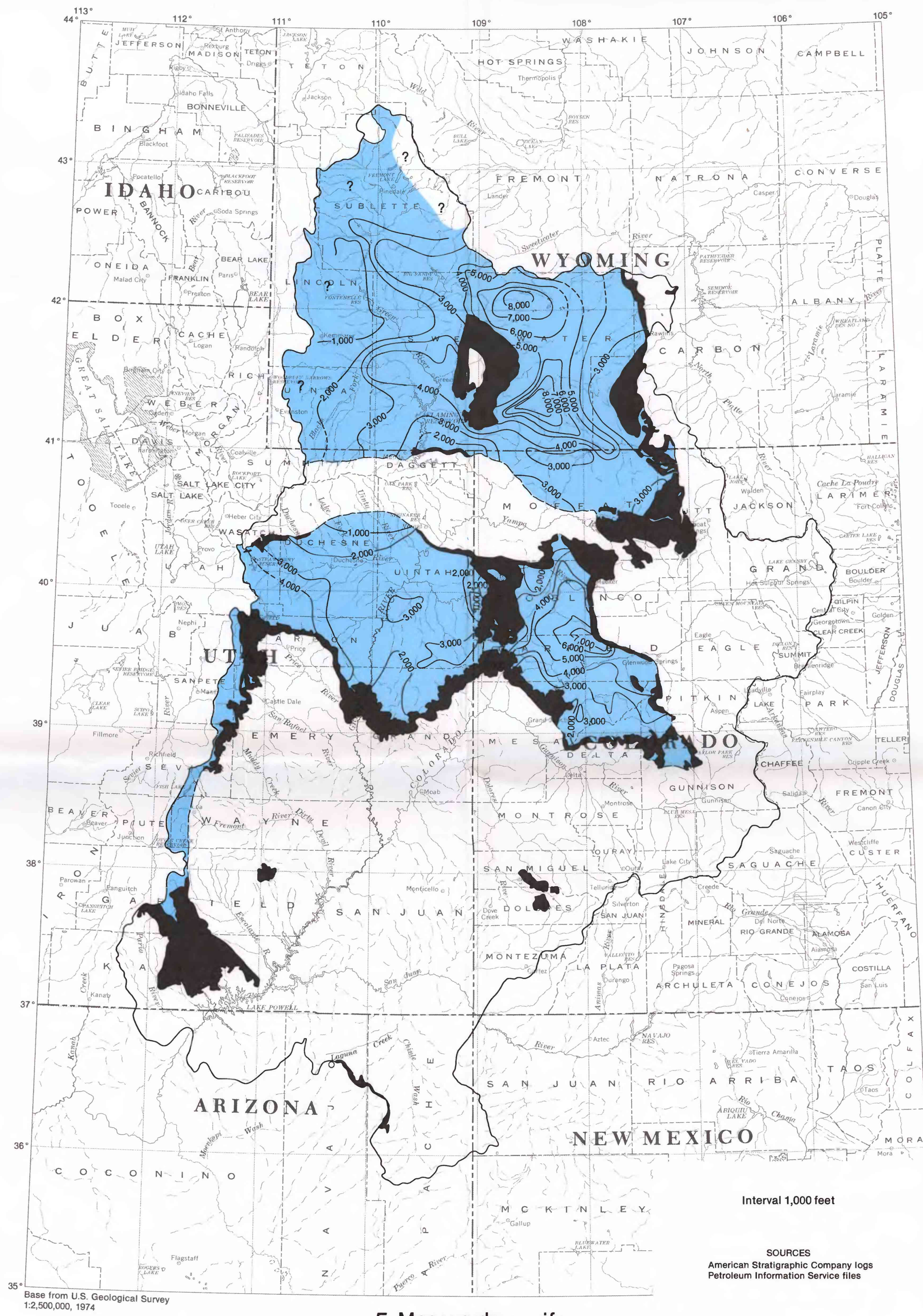
E. Mesaverde aquifer
