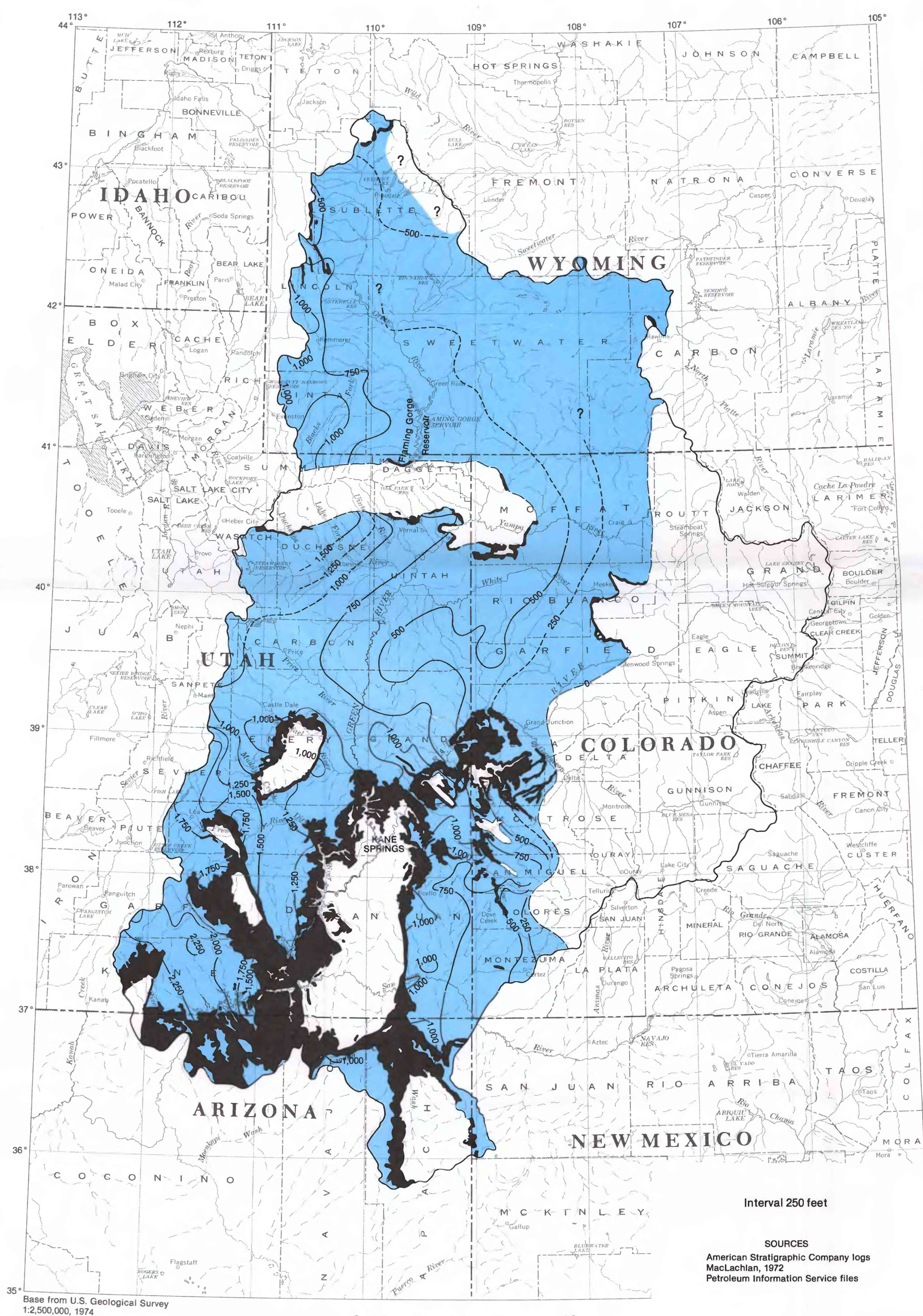
A. Navajo-Nugget aquifer
