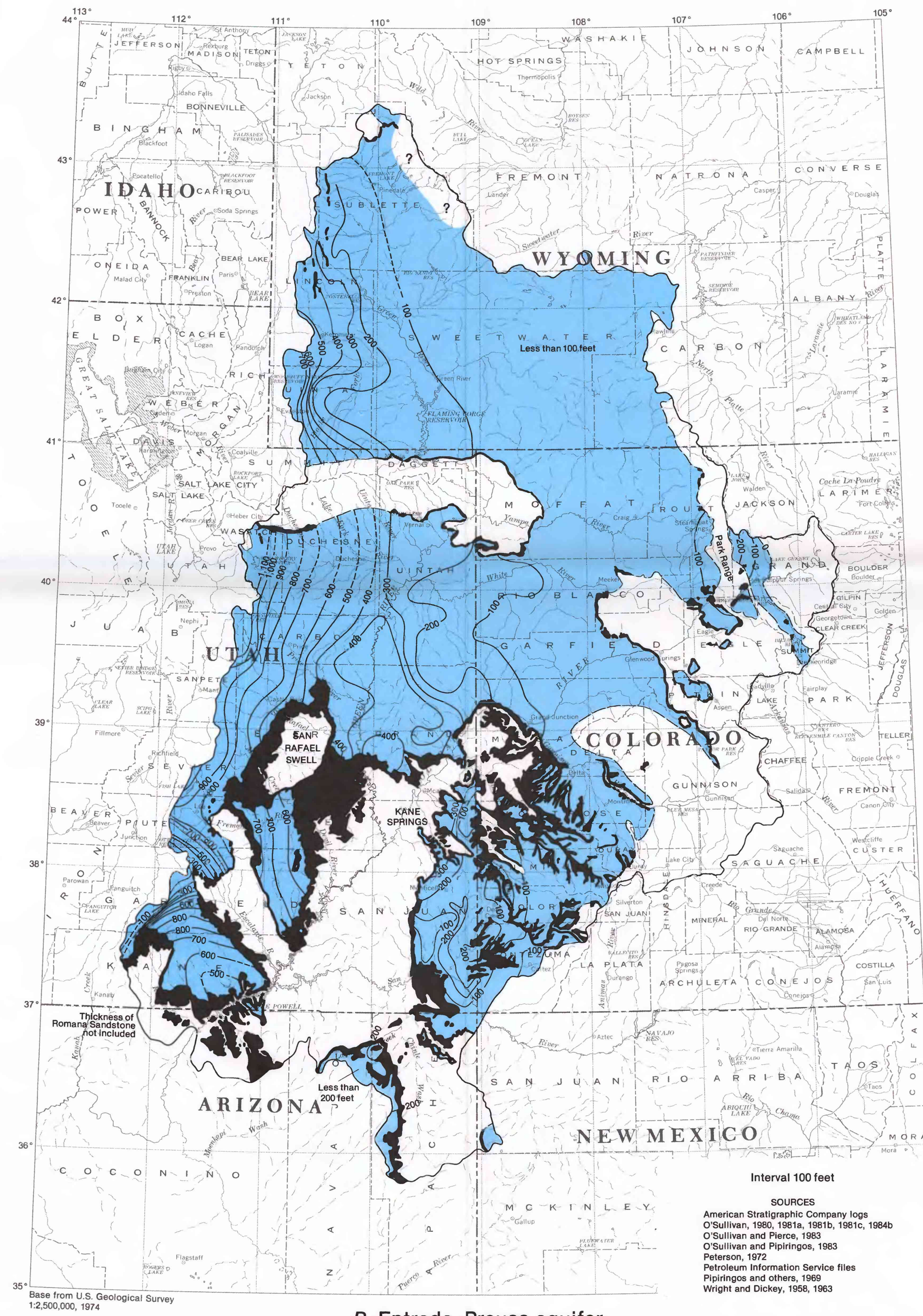
B. Entrada-Preuss aquifer
