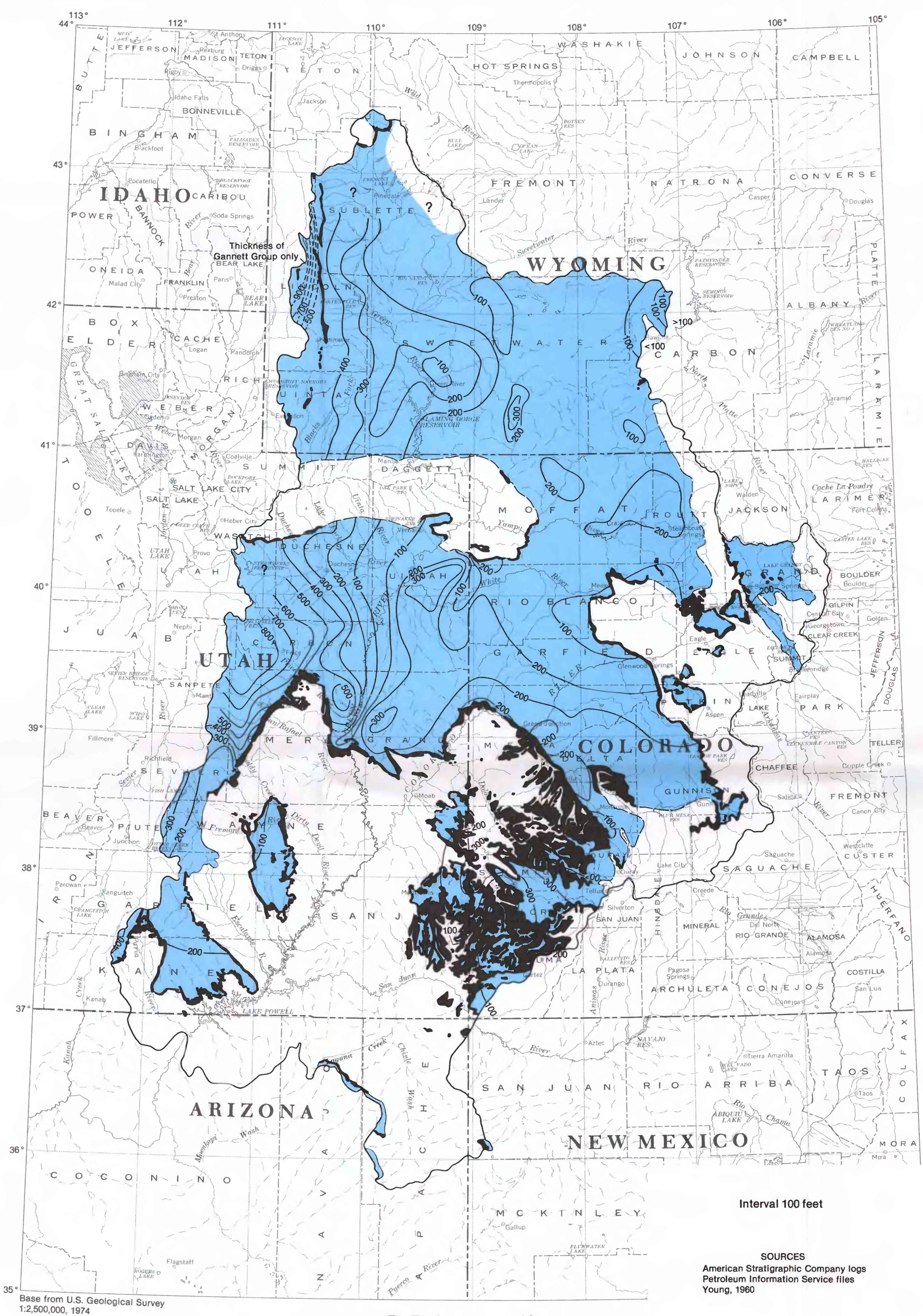
D. Dakota aquifer
