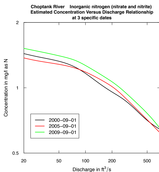
(b) plotConcQSmooth(logScale=TRUE)
