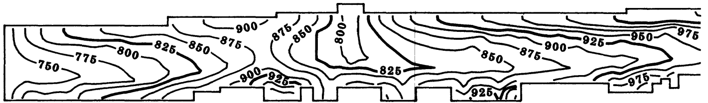
LAYER 2
