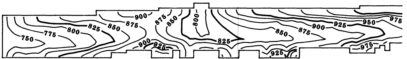
LAYER 3
