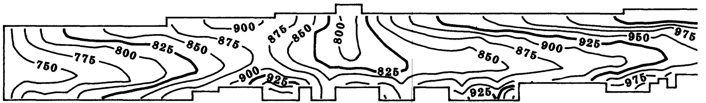
LAYER 4
