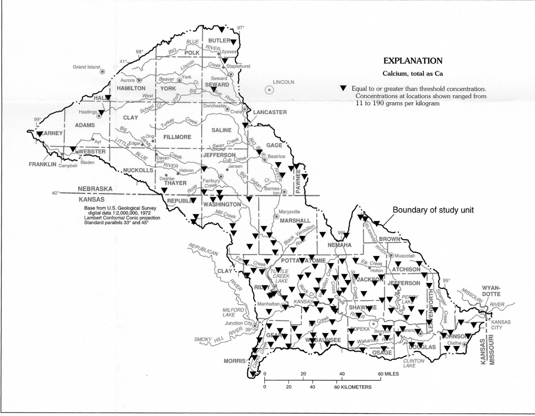
D.--Calcium
