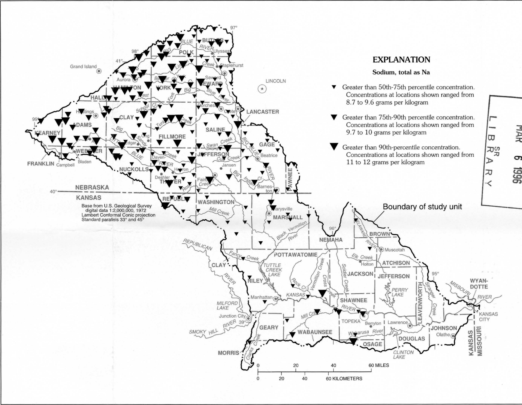
B.--Sodium
