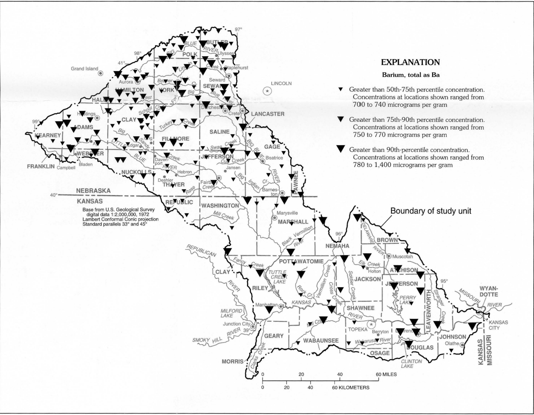
C.--Barium
