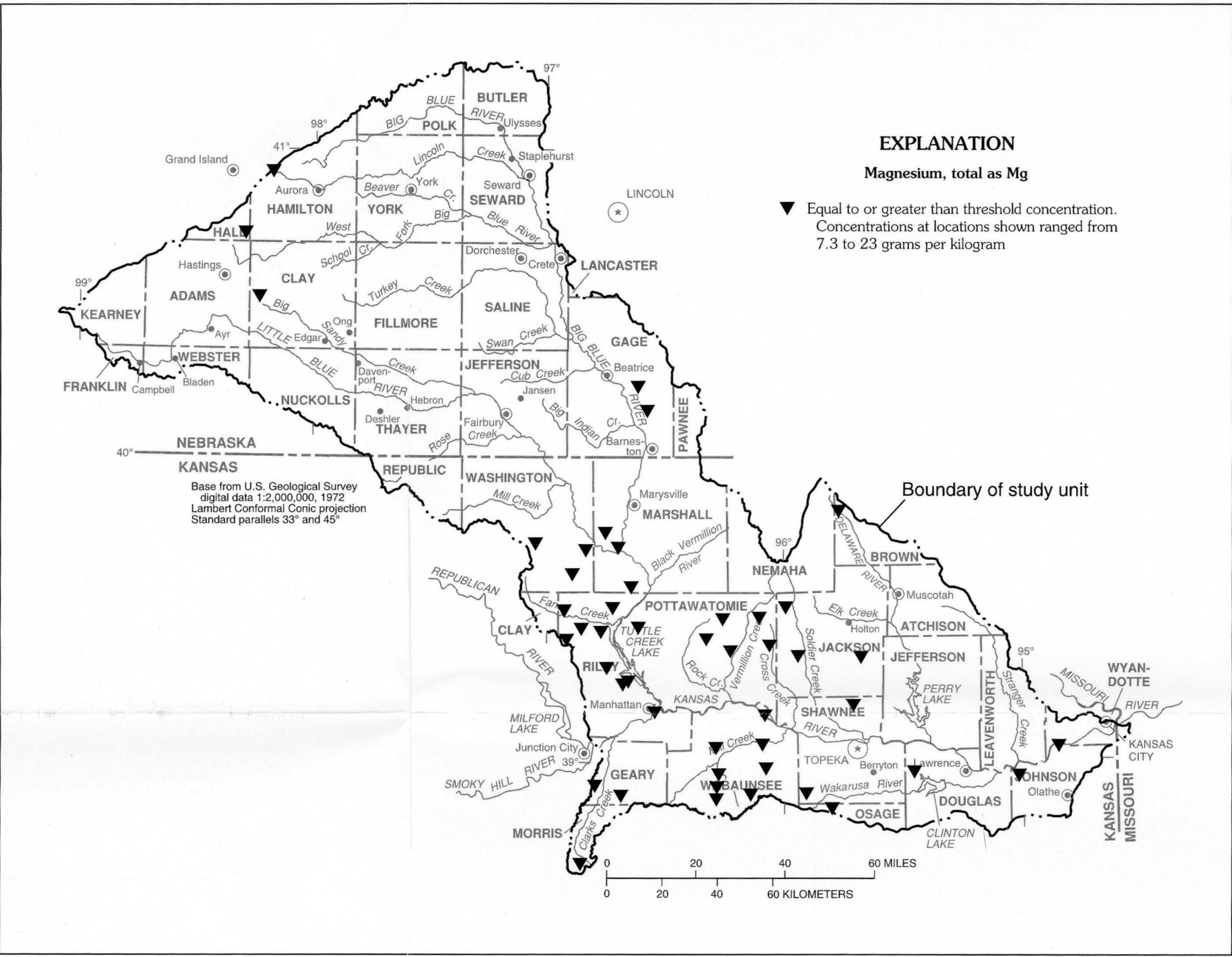
E.--Magnesium
