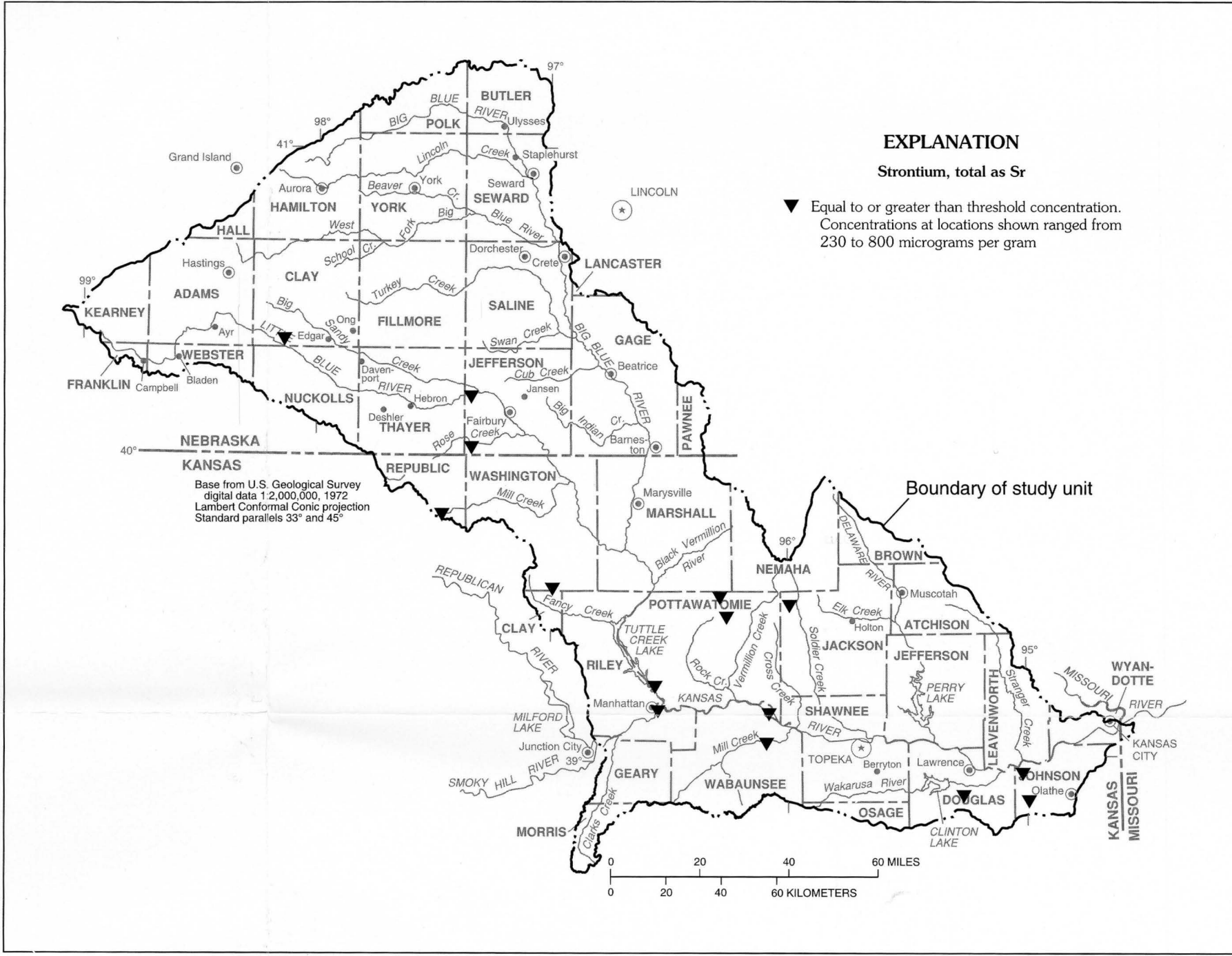
F.--Strontium
