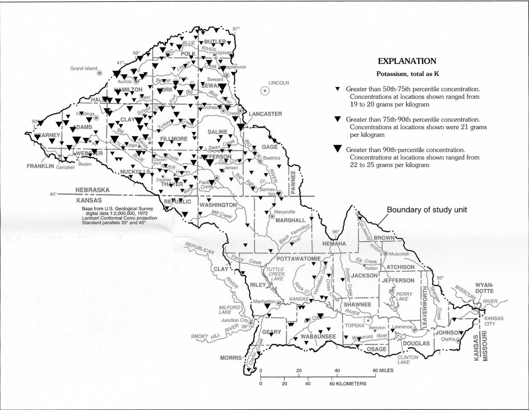
A.--Potassium
