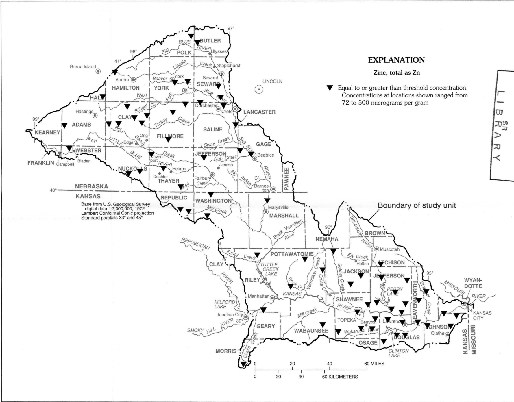
B.--Zinc
