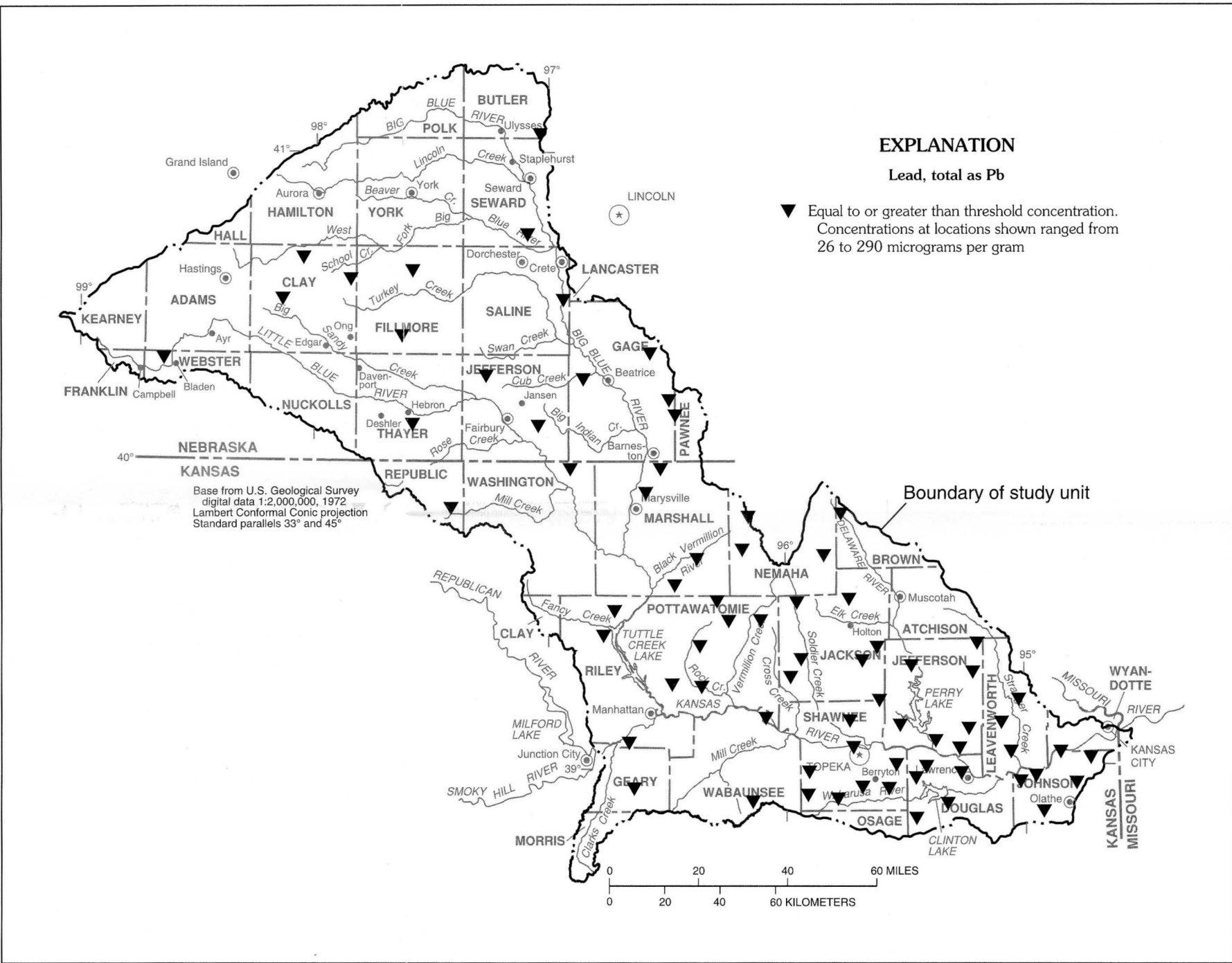
A.--Lead
