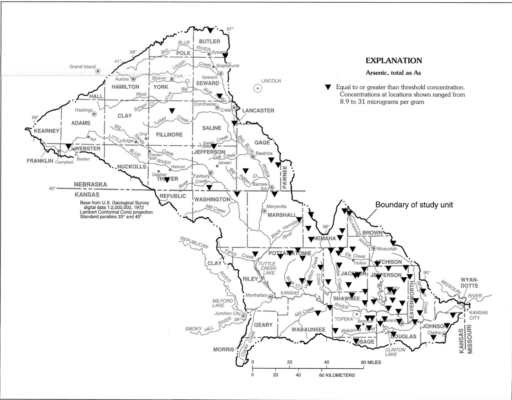
C.--Arsenic
