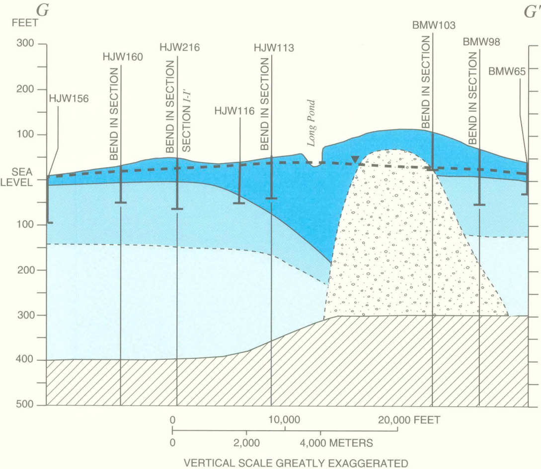
G. Hydrogeologic section G-G'
